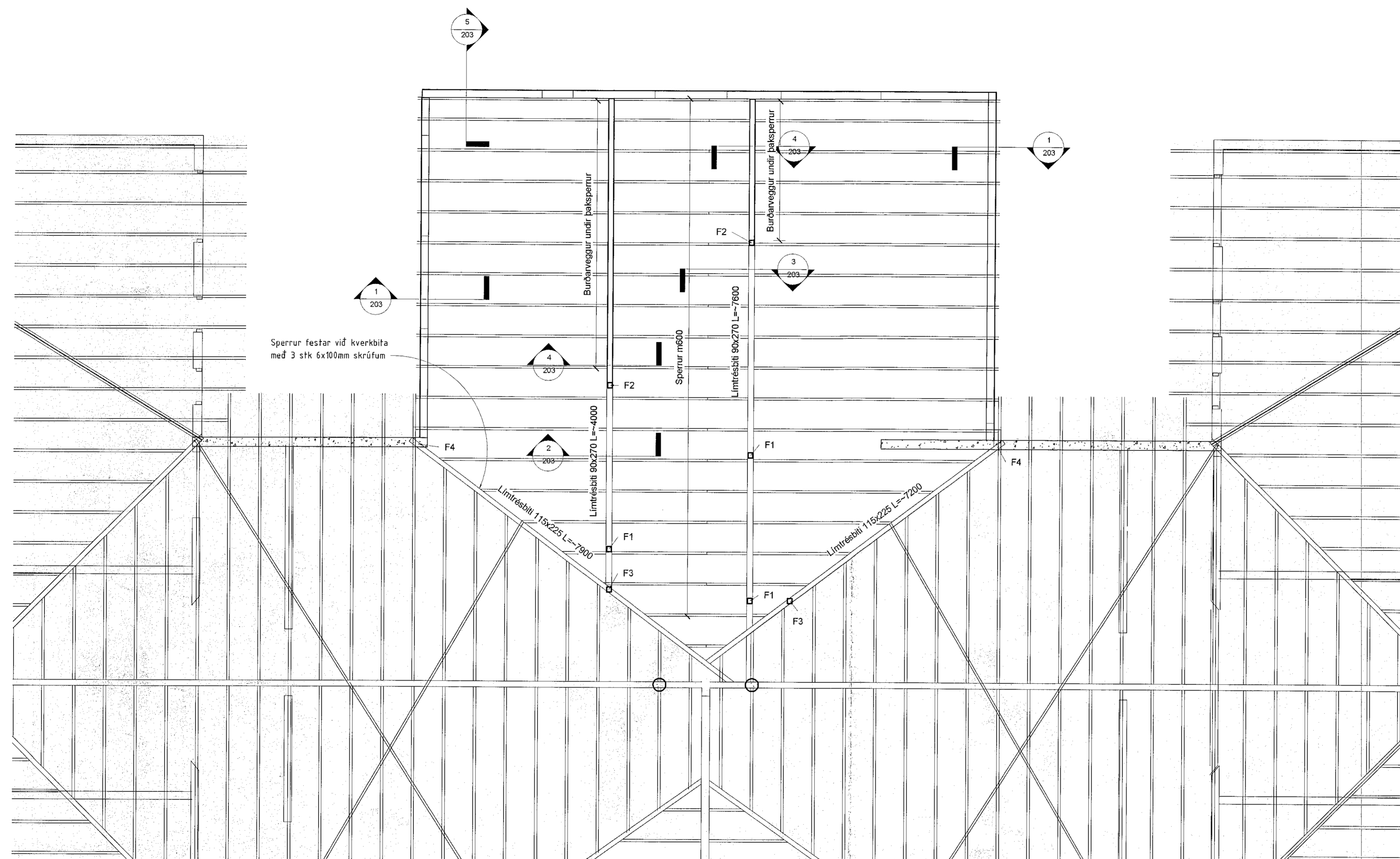
1 Þak - Grunnmynd 1 : 50
