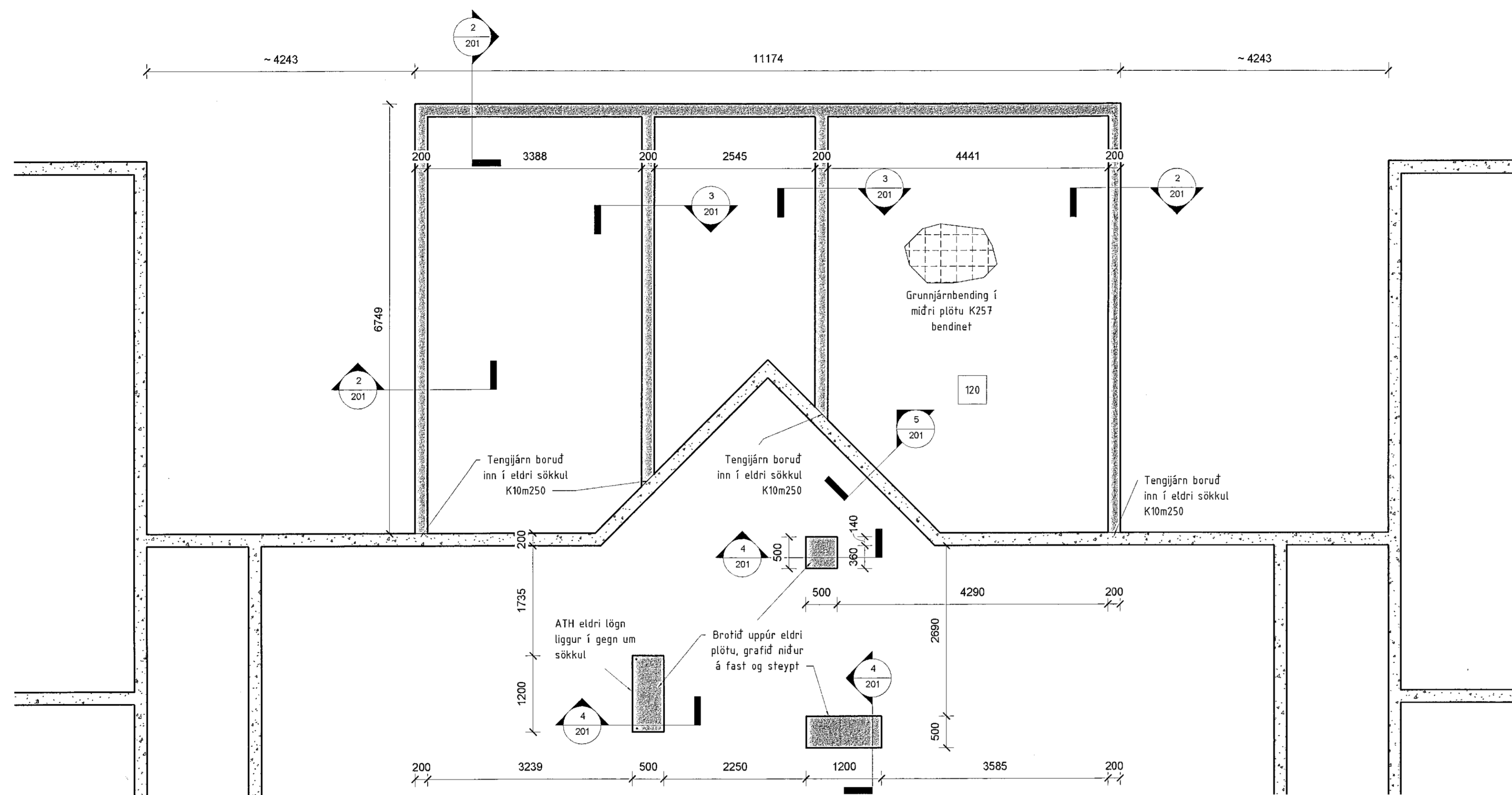
1 Grunnmynd - Viðbygging 1:50
