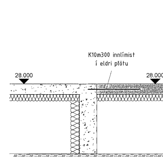
5 Snið 1:20
