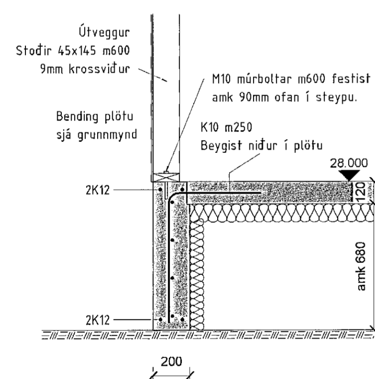
2 Snið 1:20
