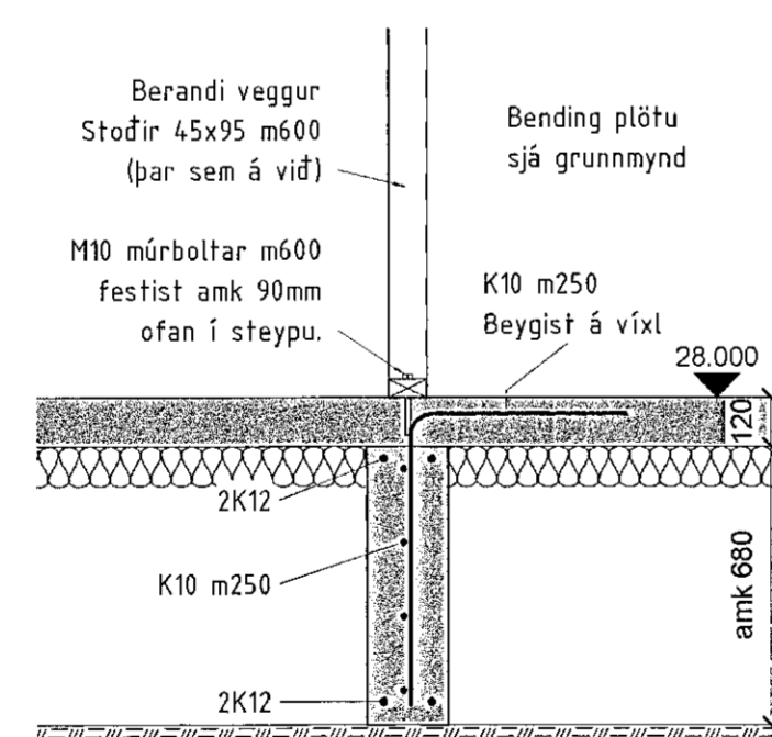
3 Snið 1:20
