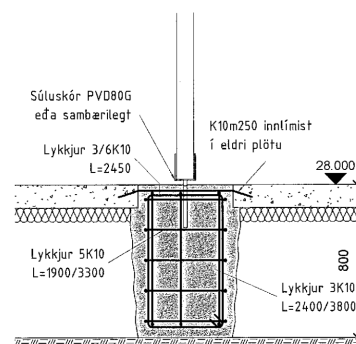
4 Snið 1:20
