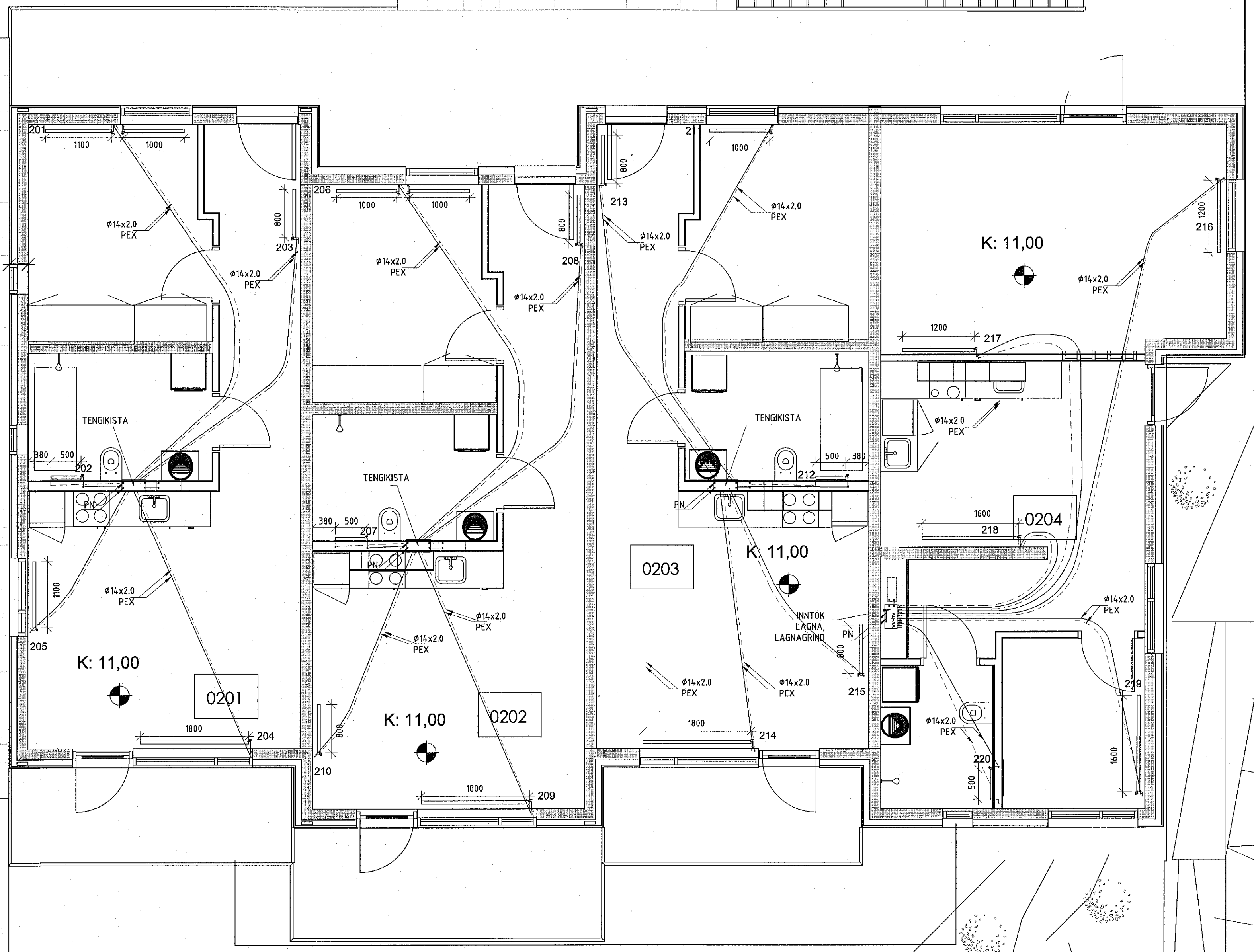
GRUNNMYND OFNALAGNIR 2.HÆÐ 1:50
