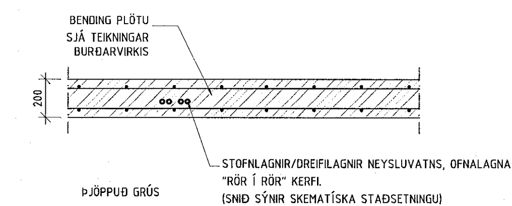
ALMENNT SNIÐ Í MILLIPLÖTU 1:20
