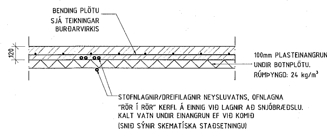
ALMENNT SNIÐ Í BÖTNPLÖTU 1:20
