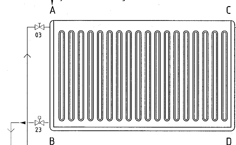
Tengimynd ofna: Stýring m. vatnshitastýrðum bakrásarloka
