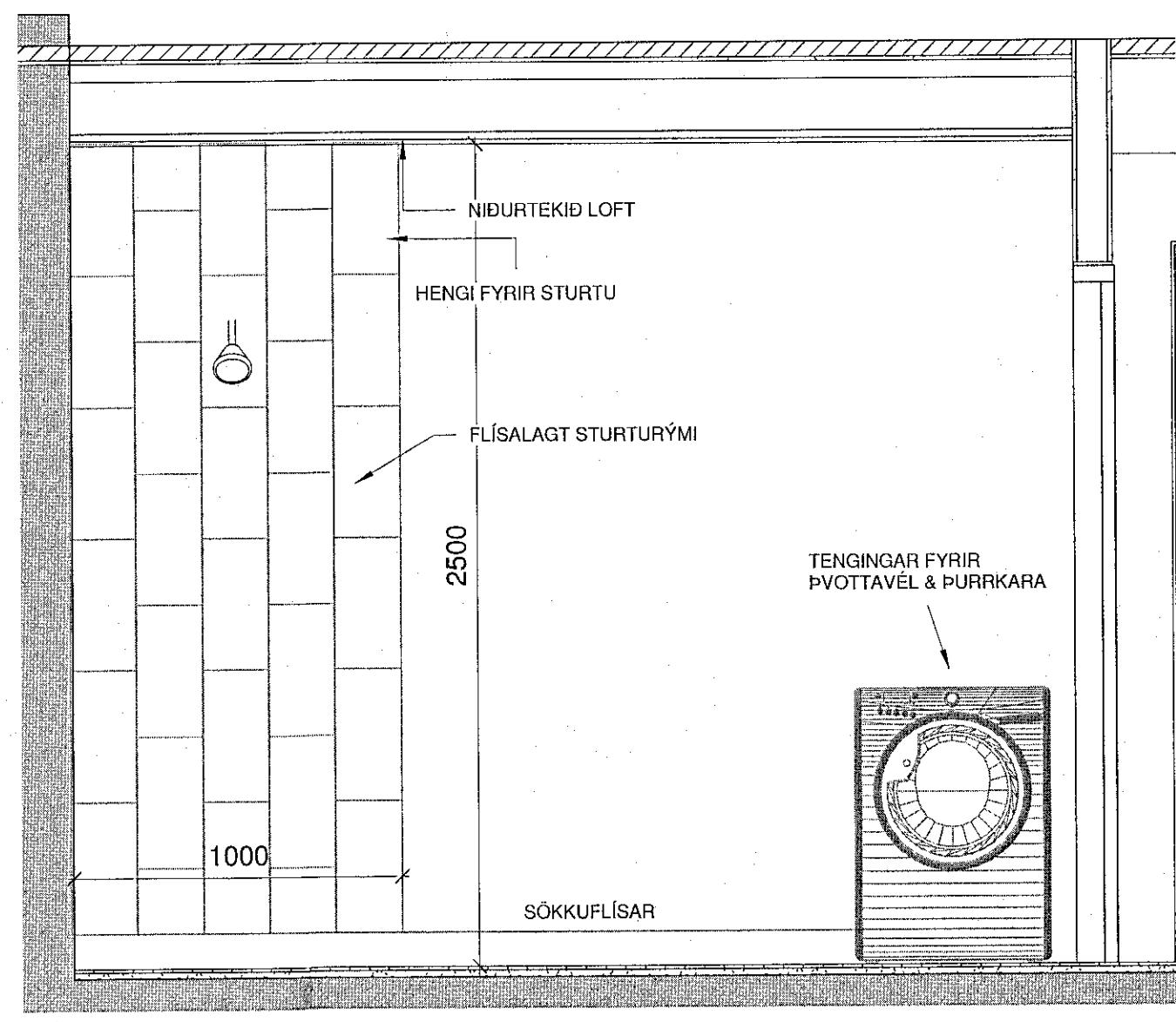
ÁSÝND BADHERBERGI_A NORÐUR VEGGUR 1:20
