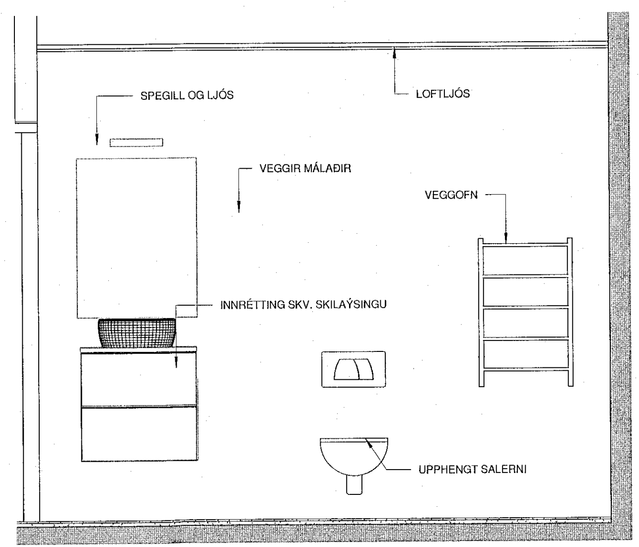
ÁSÝND BADHERBERGI_A SUÐURVEGGUR 1:20
