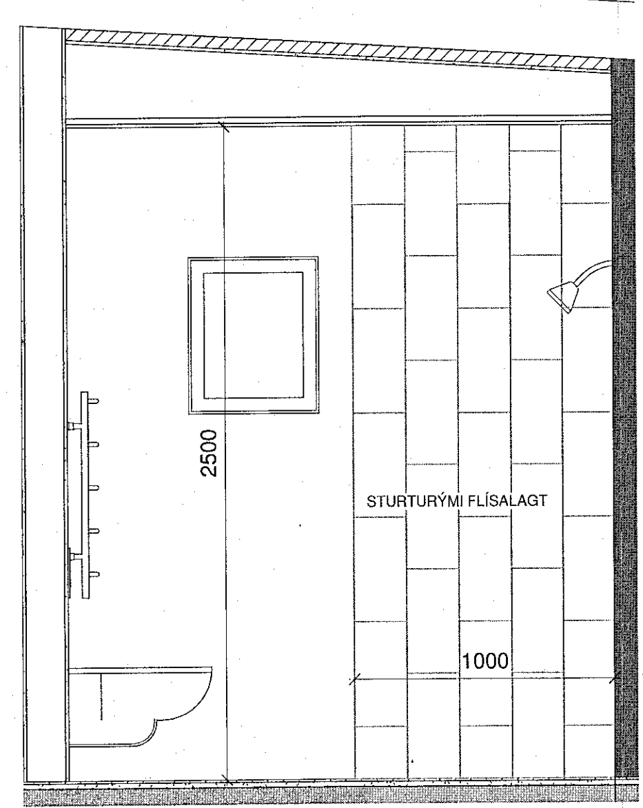
ÁSÝND BADHERBERGI_A VESTURVEGGUR 1:20
