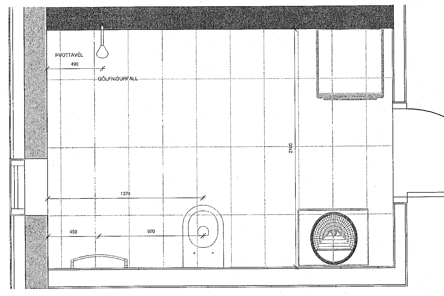
GRUNNMÝND-BADHERBERGI - HEFDBUNDIÐ A 1:20
