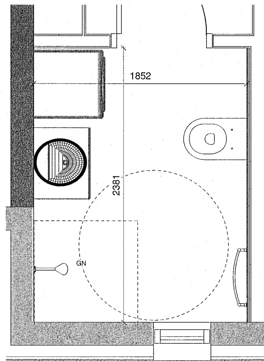
GRUNNMYND BADHERBERGI STARFSFÓLK 1 : 20
