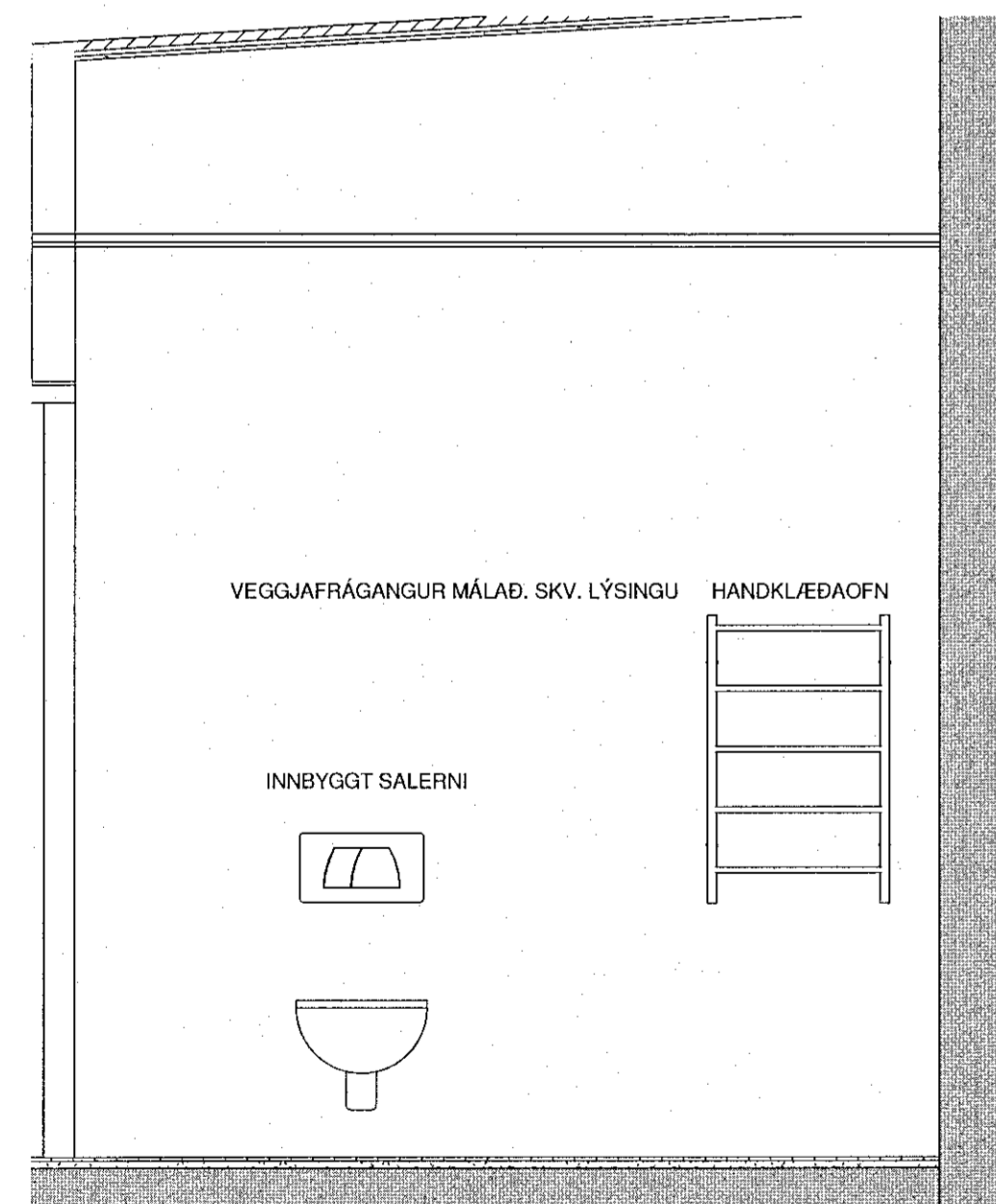
ÁSÝND BADHERBERGI_C AUSTUR 1 : 20
