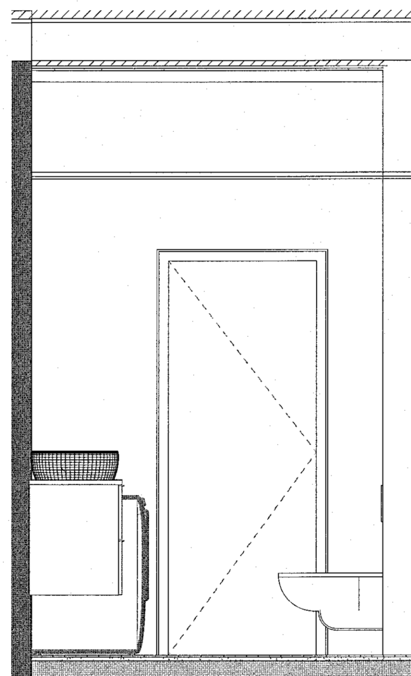
ÁSÝND BADHERBERGI_C NORÐUR 1 : 20
