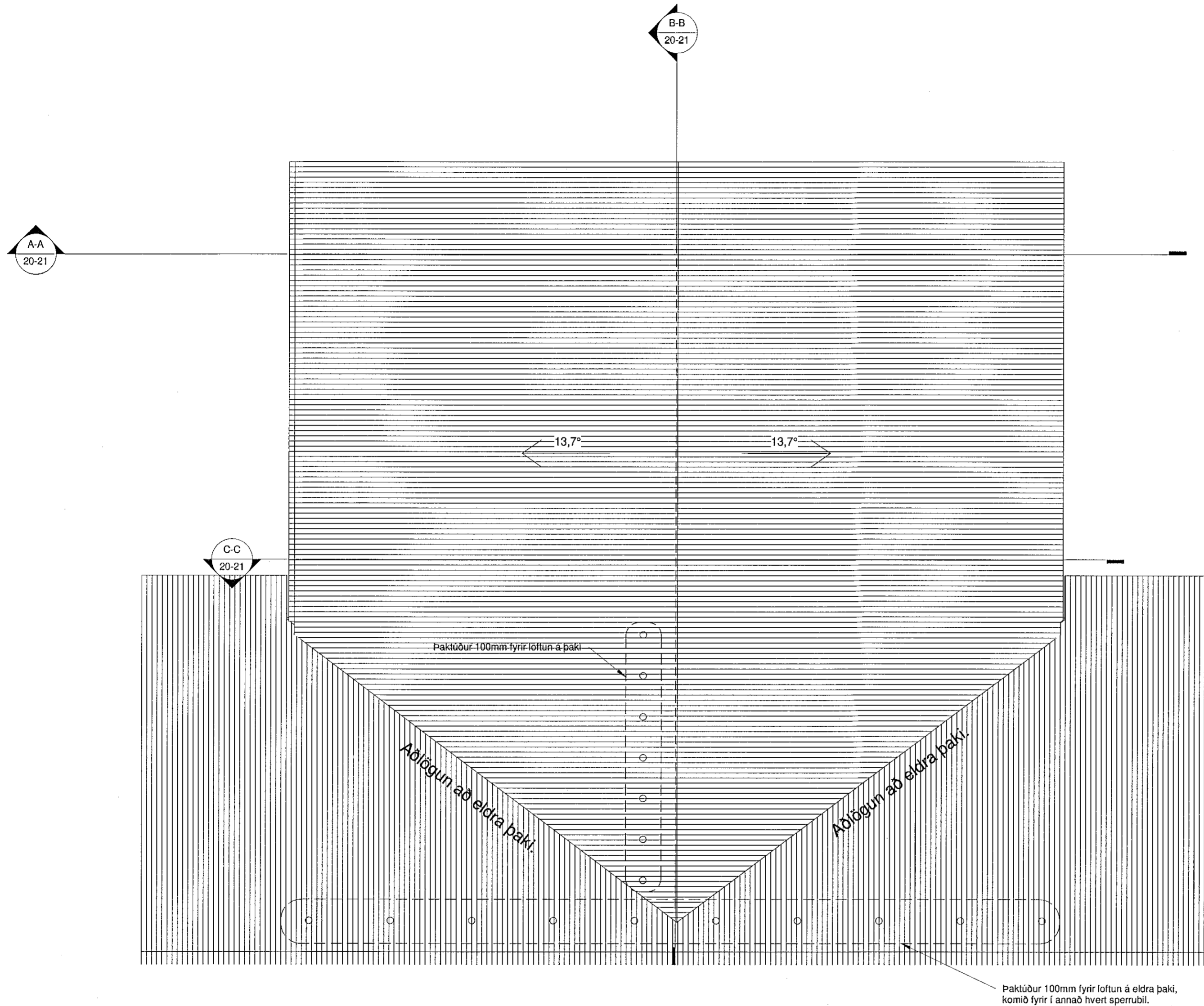
Þakmynd 1 : 50
