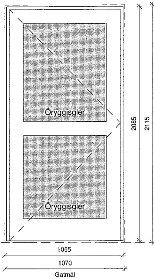
EW-30 CS H01 (1 stk.) Eldvarnarhurð
