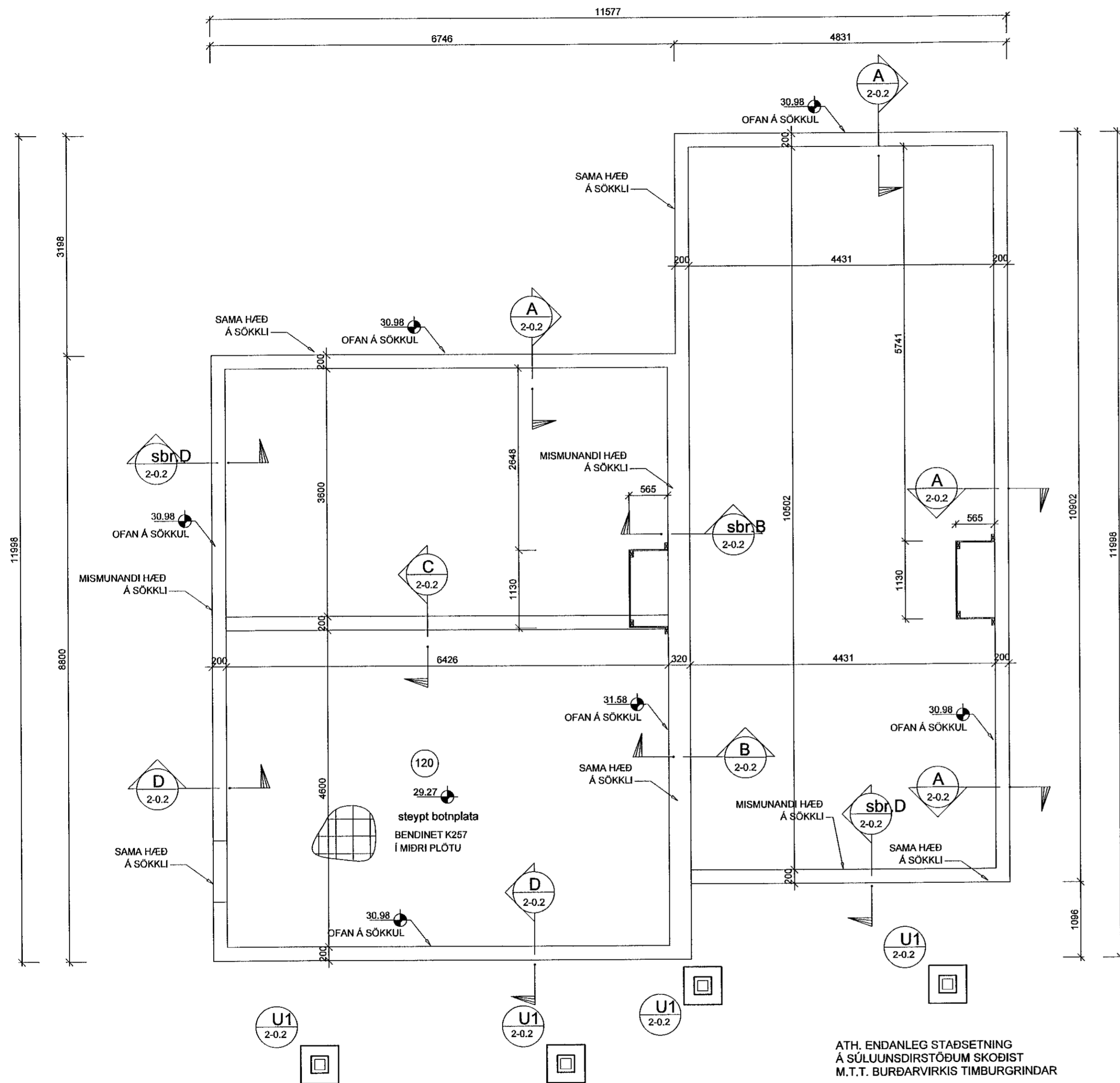
MATSHLUTI 03. GRUNNMYND SÖKKLA 1:50
