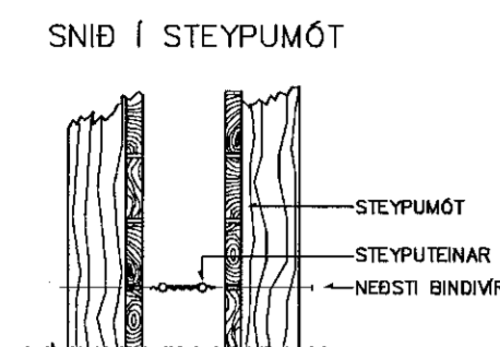
FRÁGANGUR Á SAMTENGINGUM STEYPUENA FYRIR SÖKKULJARÐSKAUT
