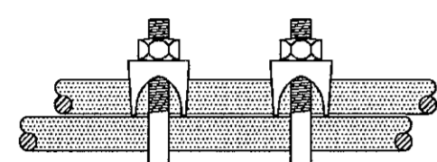
FRÁGANGUR Á SAMTENGINGUM STEYPUENA FYRIR SÖKKULJARÐSKAUT
