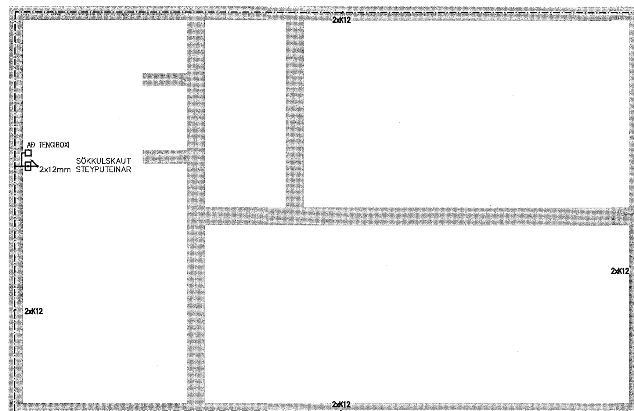
FRÁGANGUR Á SAMTENGINGUM STEYPUENA FYRIR SÖKKULJARÐSKAUT
