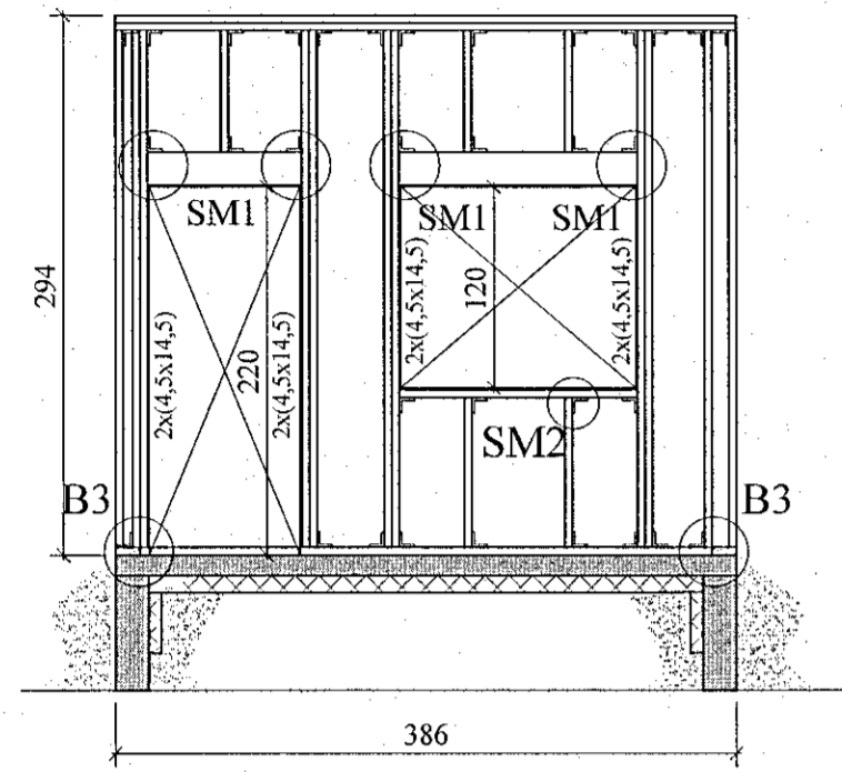
V1, VESTURHLIÐ. 1:50
