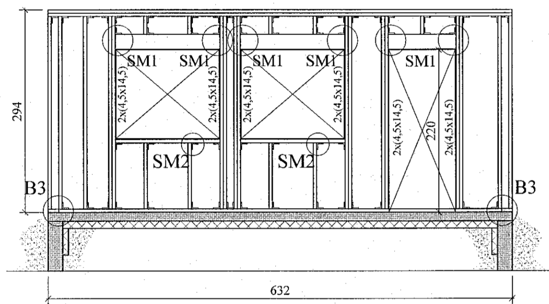
V4, SUÐURHLIÐ. 1:50
