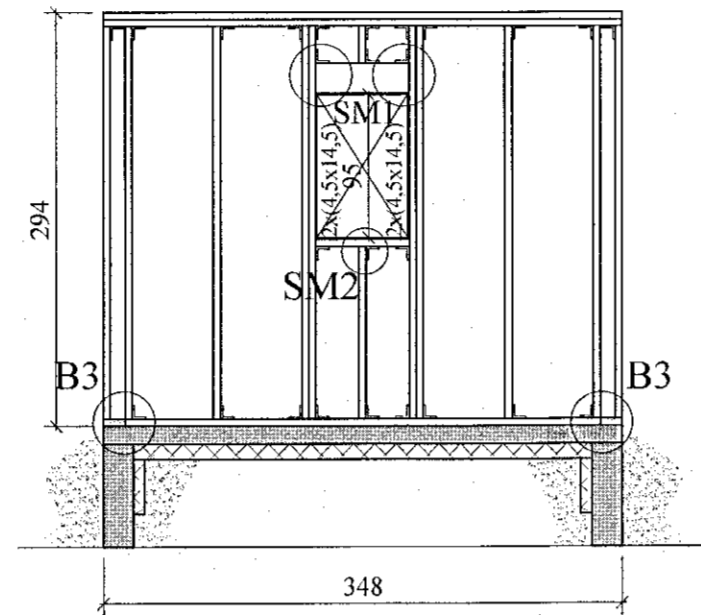
V3, VESTURHLIÐ. 1:50
