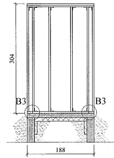
V2, NORÐURHLIÐ. 1:50
