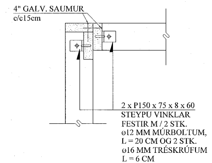
B3 SNIÐ. 1:10 1-03 ALMENNT SNIÐ Í HORNUM
