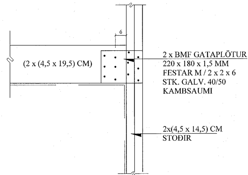
SM1 SÉRMYND. 1:10 1-03
