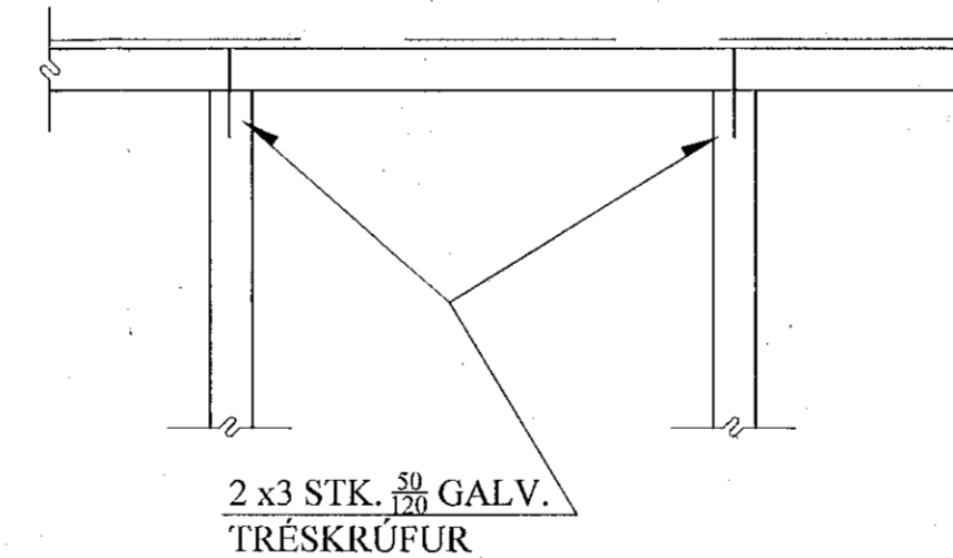
SM2 SÉRMYND. 1:10 1-03
