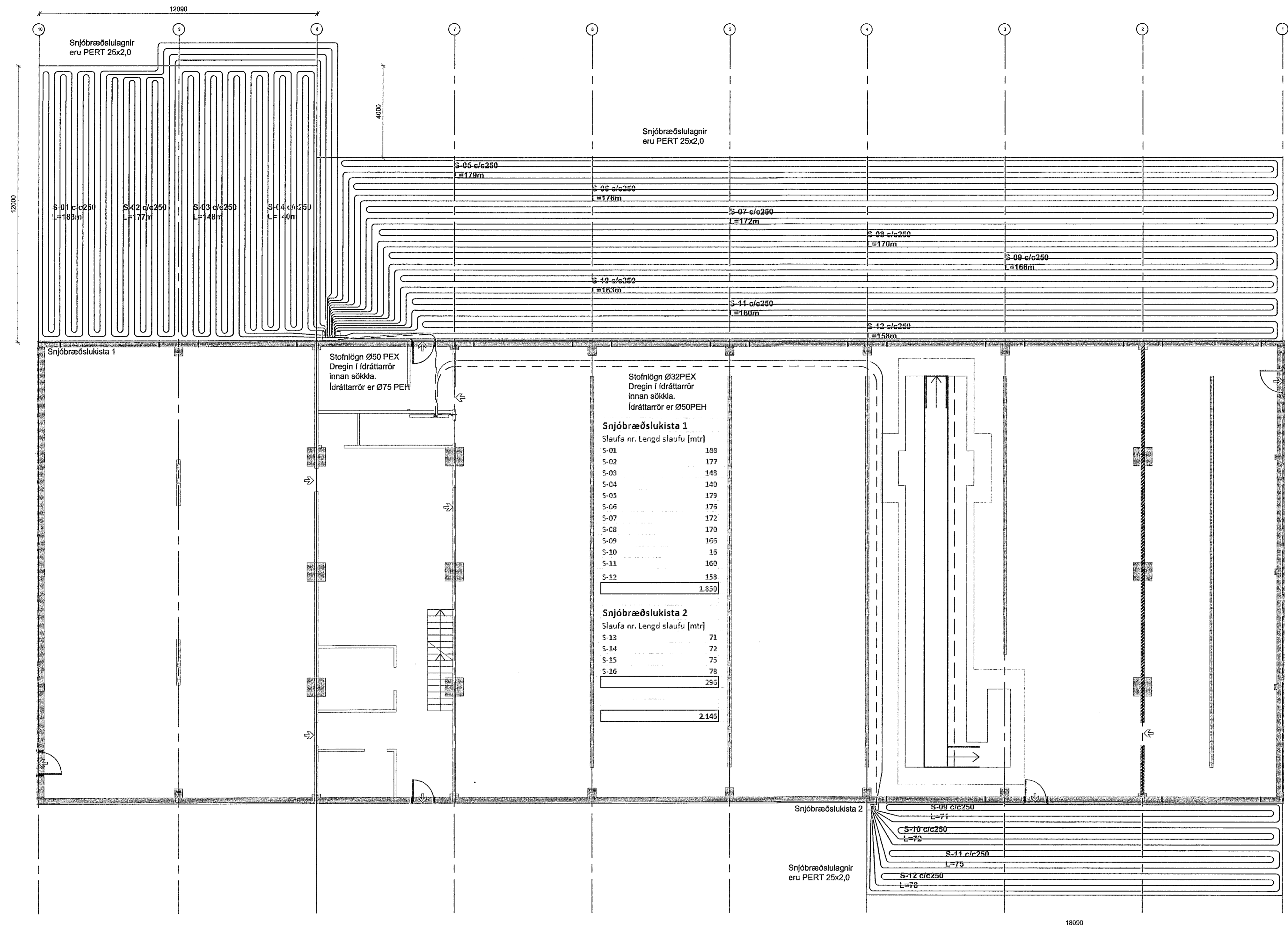
Snjóbræðsla grunnmynd M 1:100
