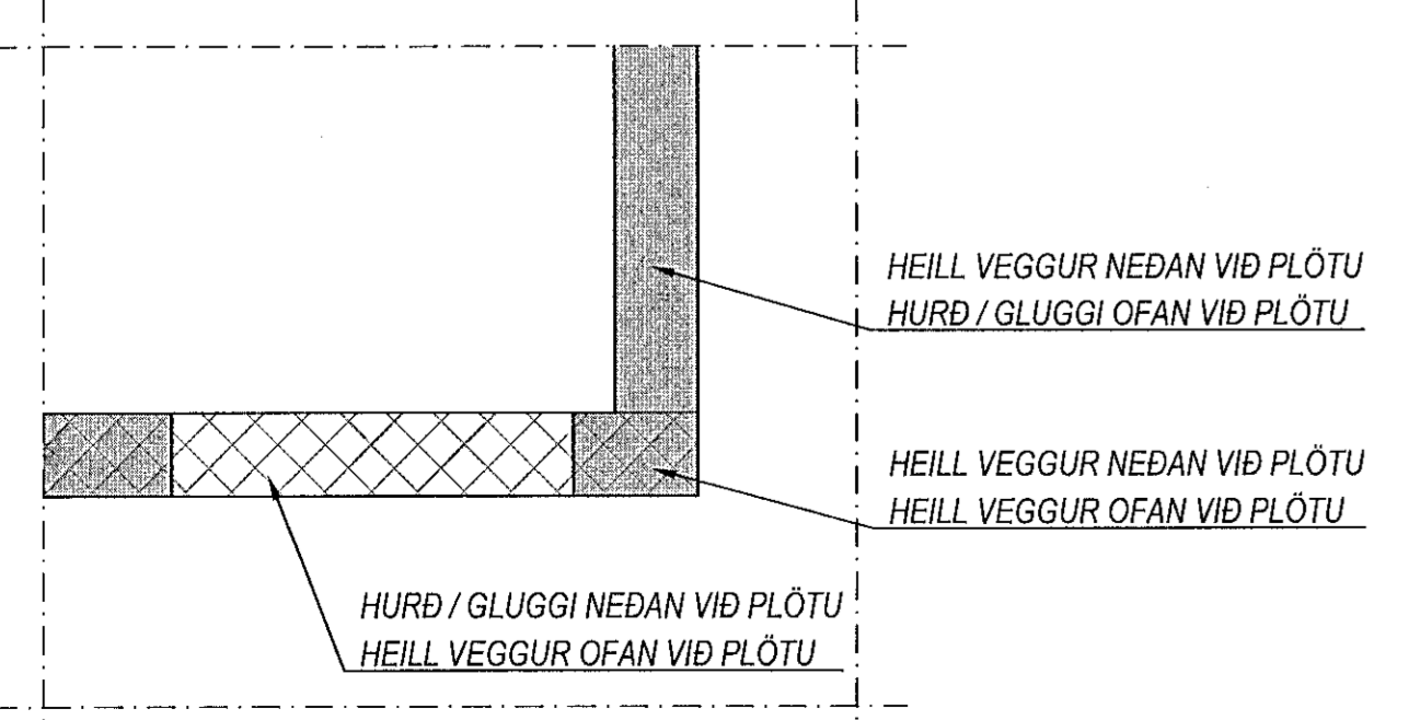
MYNSTURSTÁKN 1:20
