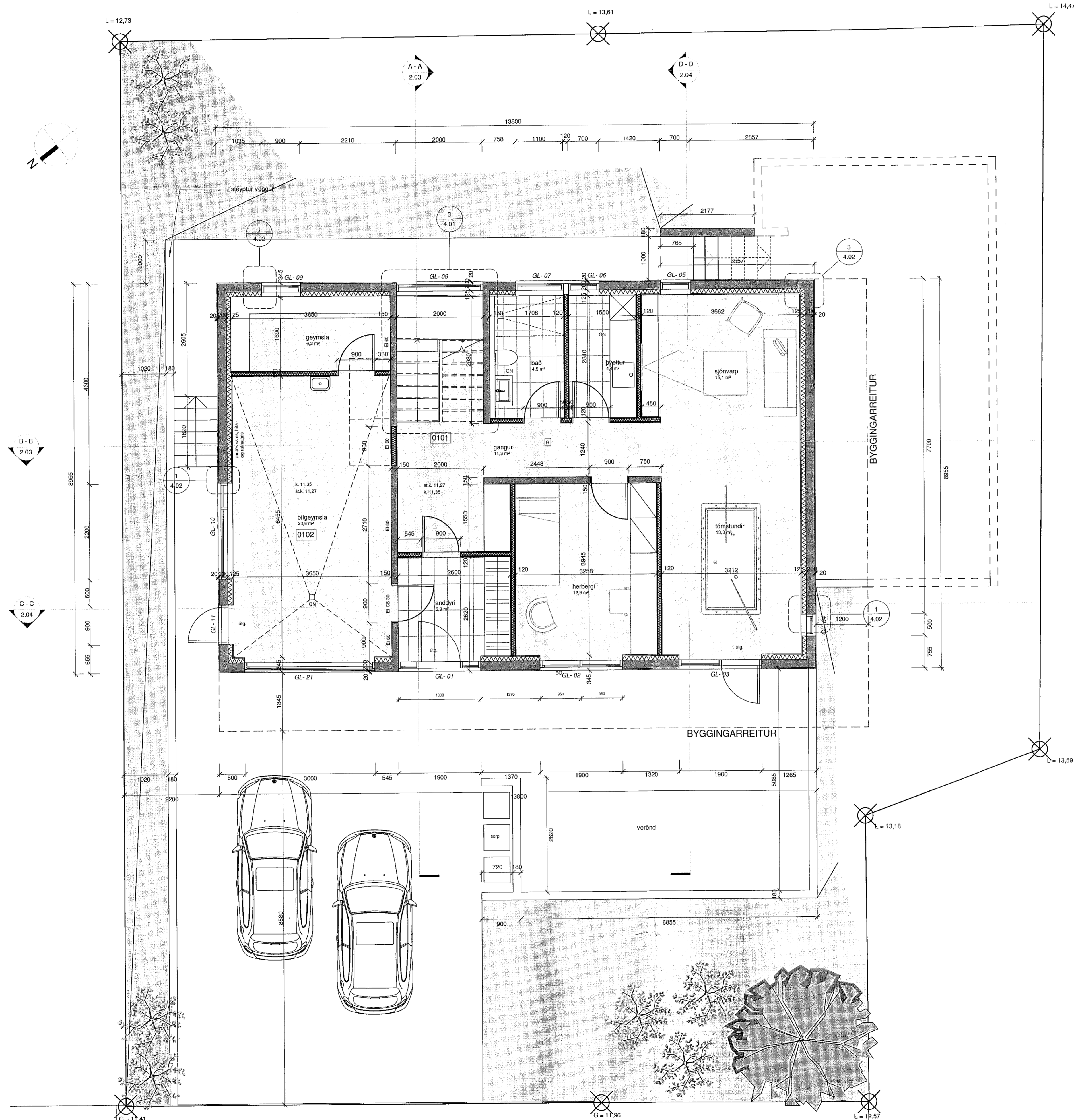
GRUNNMYND 1.HÆÐ. 1:50
