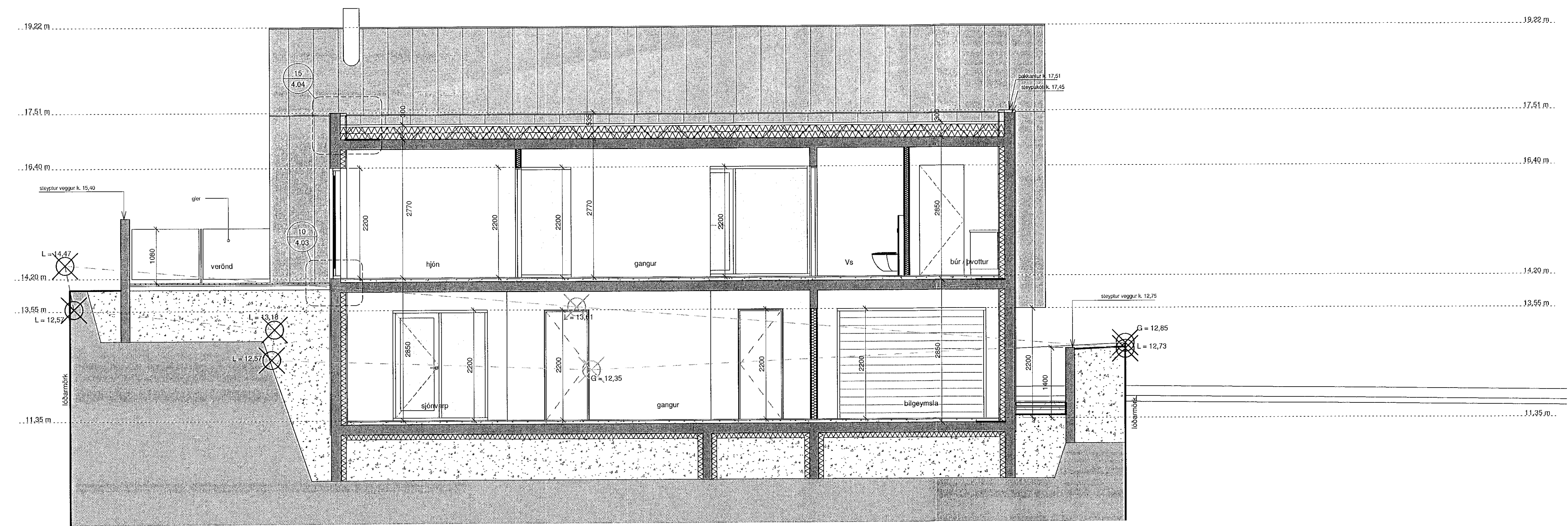
SNEIÐING B-B 1 : 50
