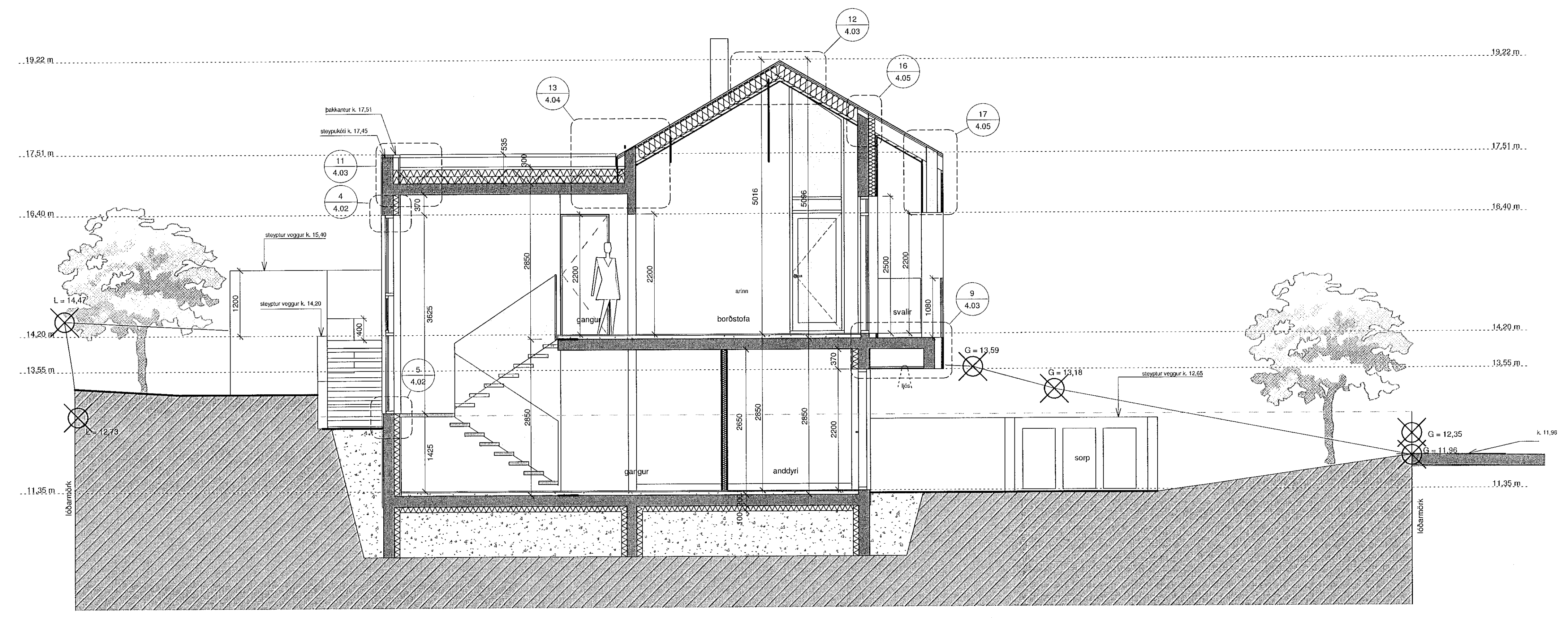
SNEIÐING A-A 1 : 50
