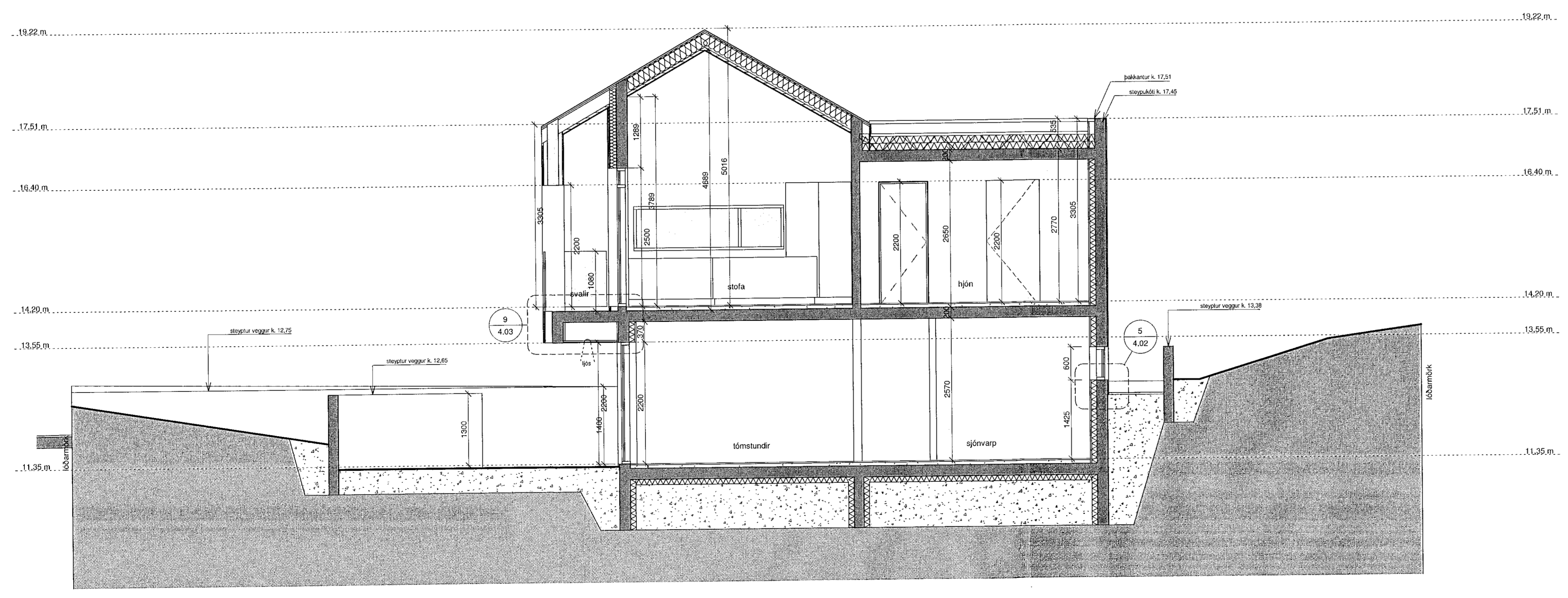
SNEIDING D-D 1:50
