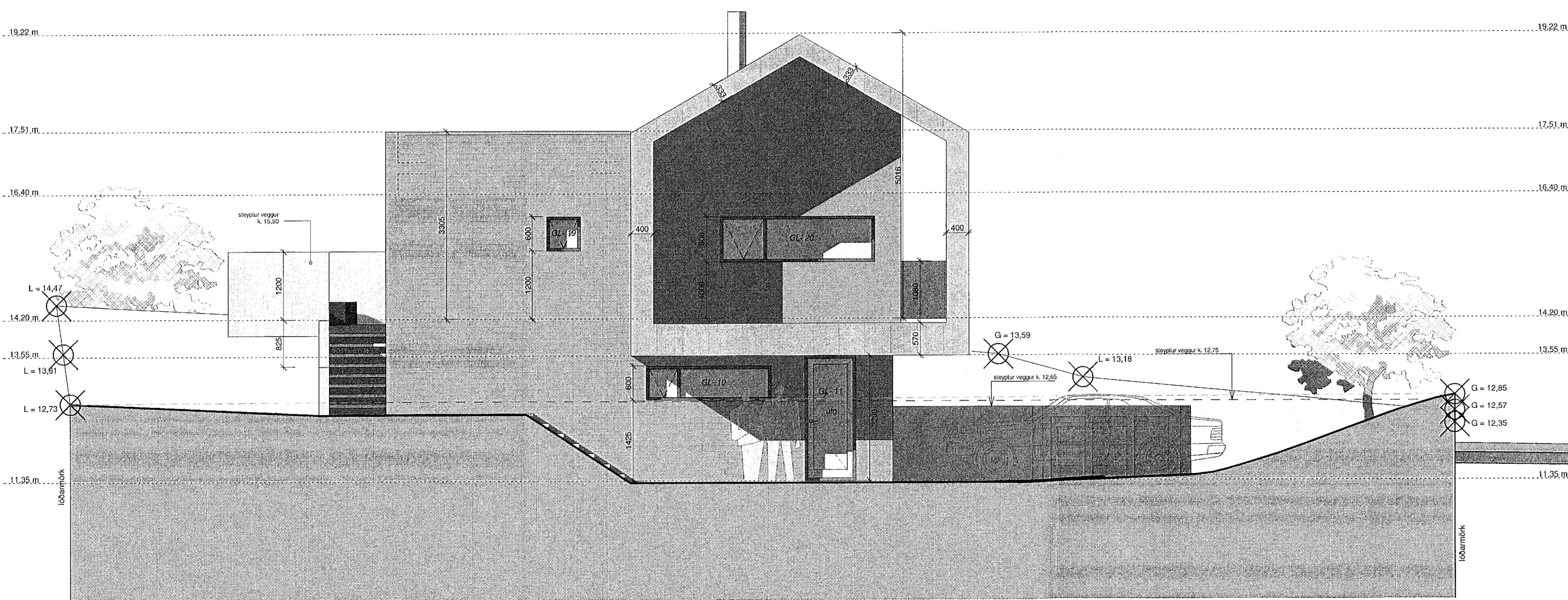
ÚTLIT NORÐAUSTUR. 1:50
