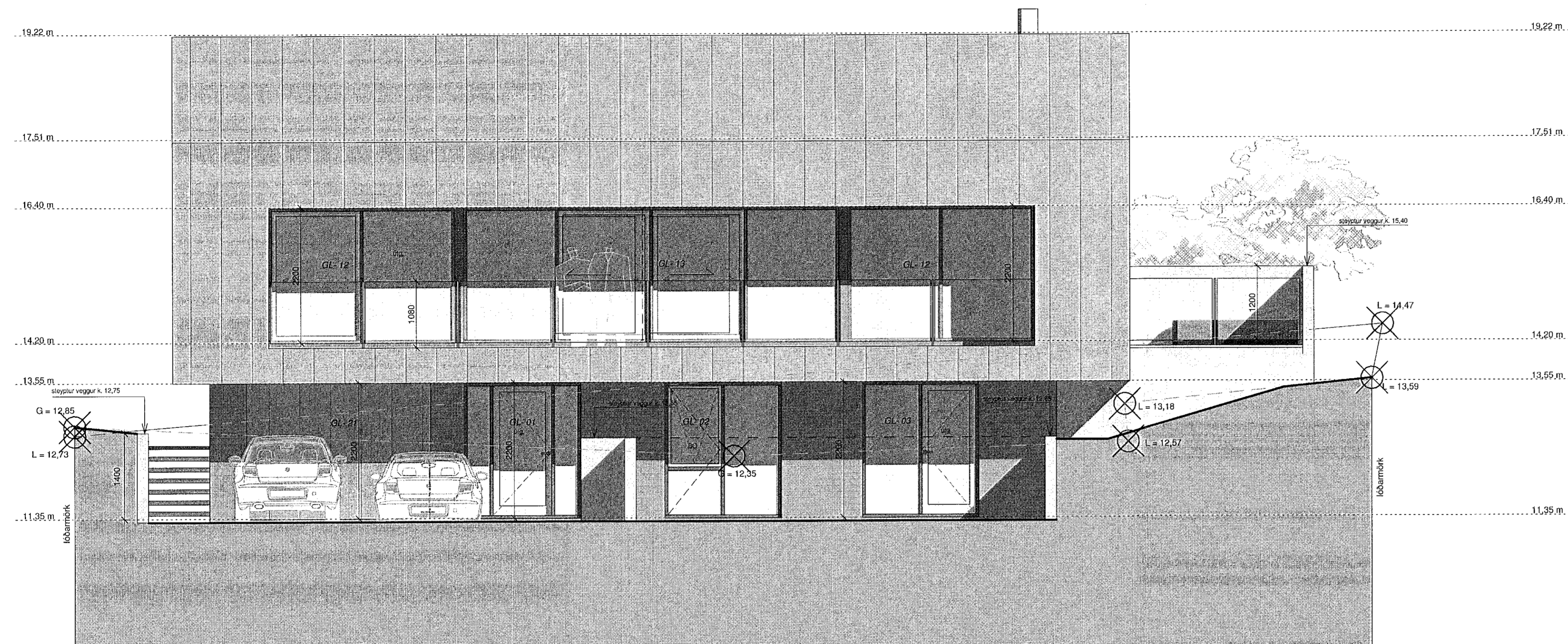
ÚTLIT NORÐVESTUR. 1:50
