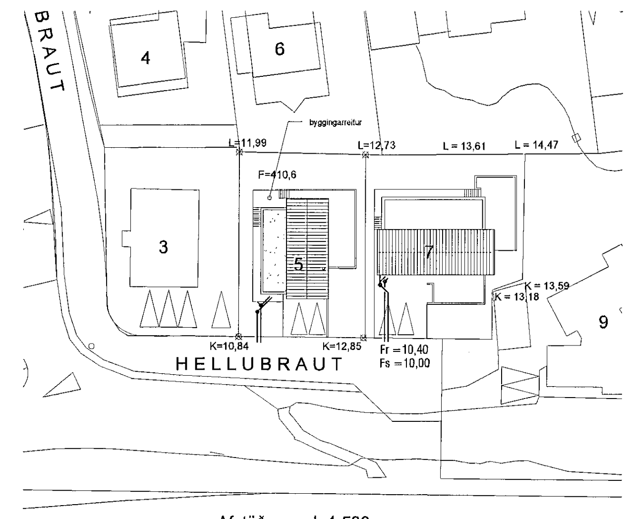
Afstöðumynd, 1:500
