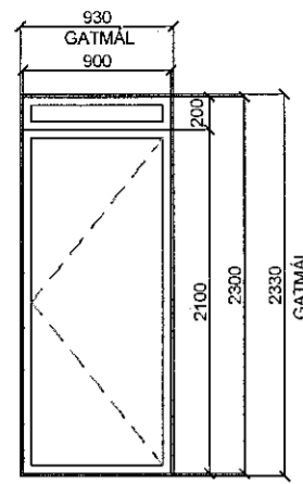
UH-01 1 STK SAMTALS ÁLTIMBURHURÐ LITIR VELJIST Í SAMRÁÐI VIÐ ARKITEKT
