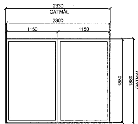
G-01 2 STK SAMTALS ÁLTIMBURGLUGGI LITIR VELJIST Í SAMRÁÐI VIÐ ARKITEKT
