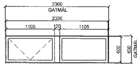
G-02 1 STK SAMTALS ÁLTIMBURGLUGGI LITIR VELJIST Í SAMRÁÐI VIÐ ARKITEKT
