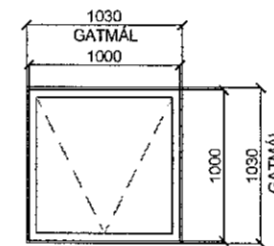
G-04 1 STK SAMTALS ÁLTIMBURGLUGGI LITIR VELJIST Í SAMRÁÐI VIÐ ARKITEKT
