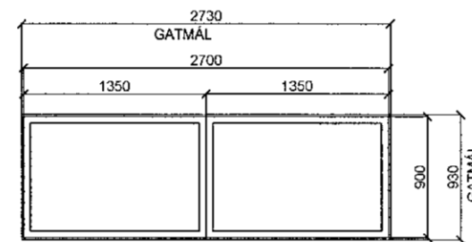
G-03 1 STK SAMTALS ÁLTIMBURGLUGGI LITIR VELJIST Í SAMRÁÐI VIÐ ARKITEKT
