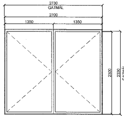
UH-02 1 STK SAMTALS ÁLTIMBURHURÐ LITIR VELJIST Í SAMRÁÐI VIÐ ARKITEKT
