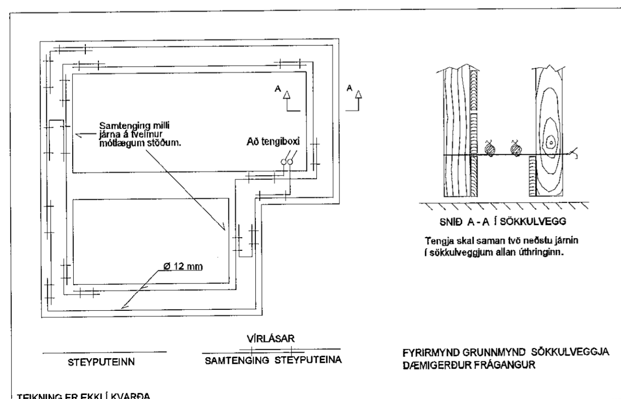
TEIKNING ER EKKI Í KVARÐA
