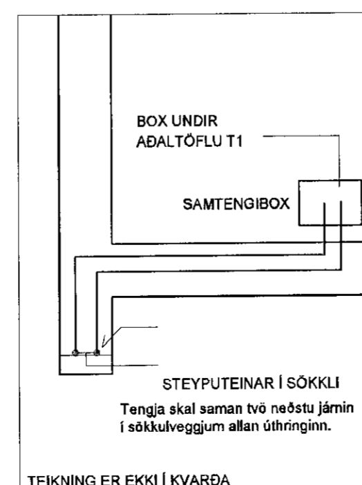
TEIKNING ER EKKI Í KVARÐA
