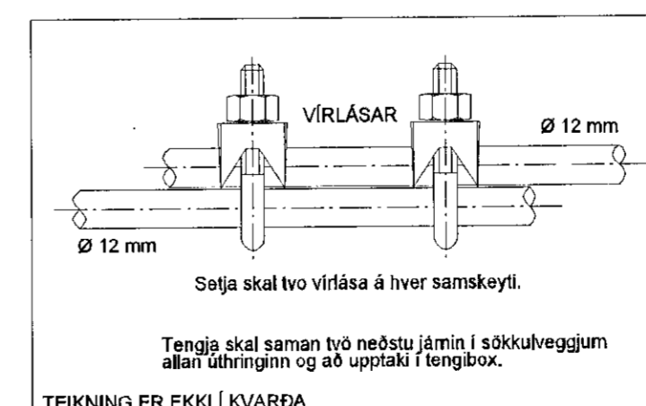
TEIKNING ER EKKI Í KVARÐA
