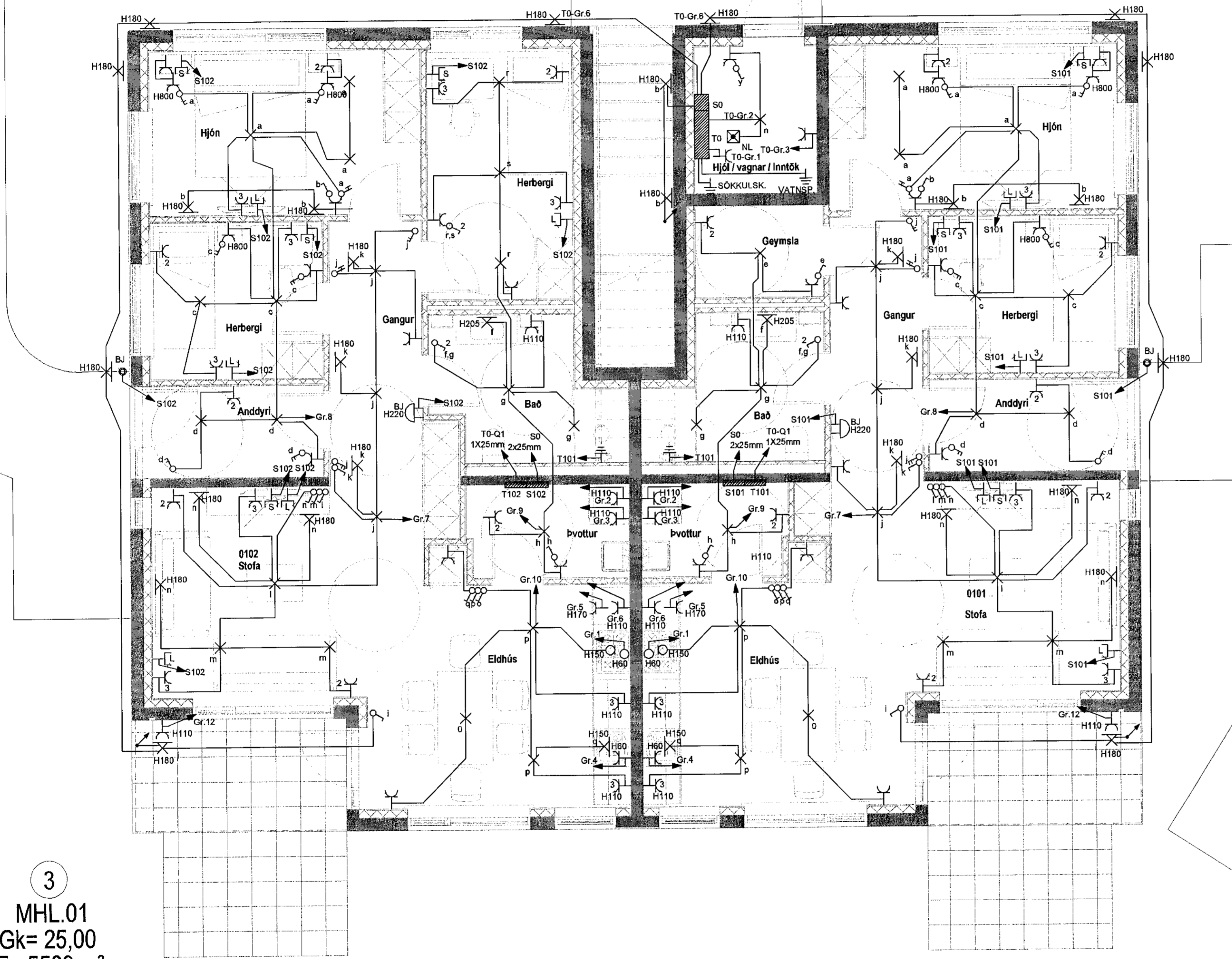
GRUNNMYND 1.HÆÐ Mkv. 1:50
