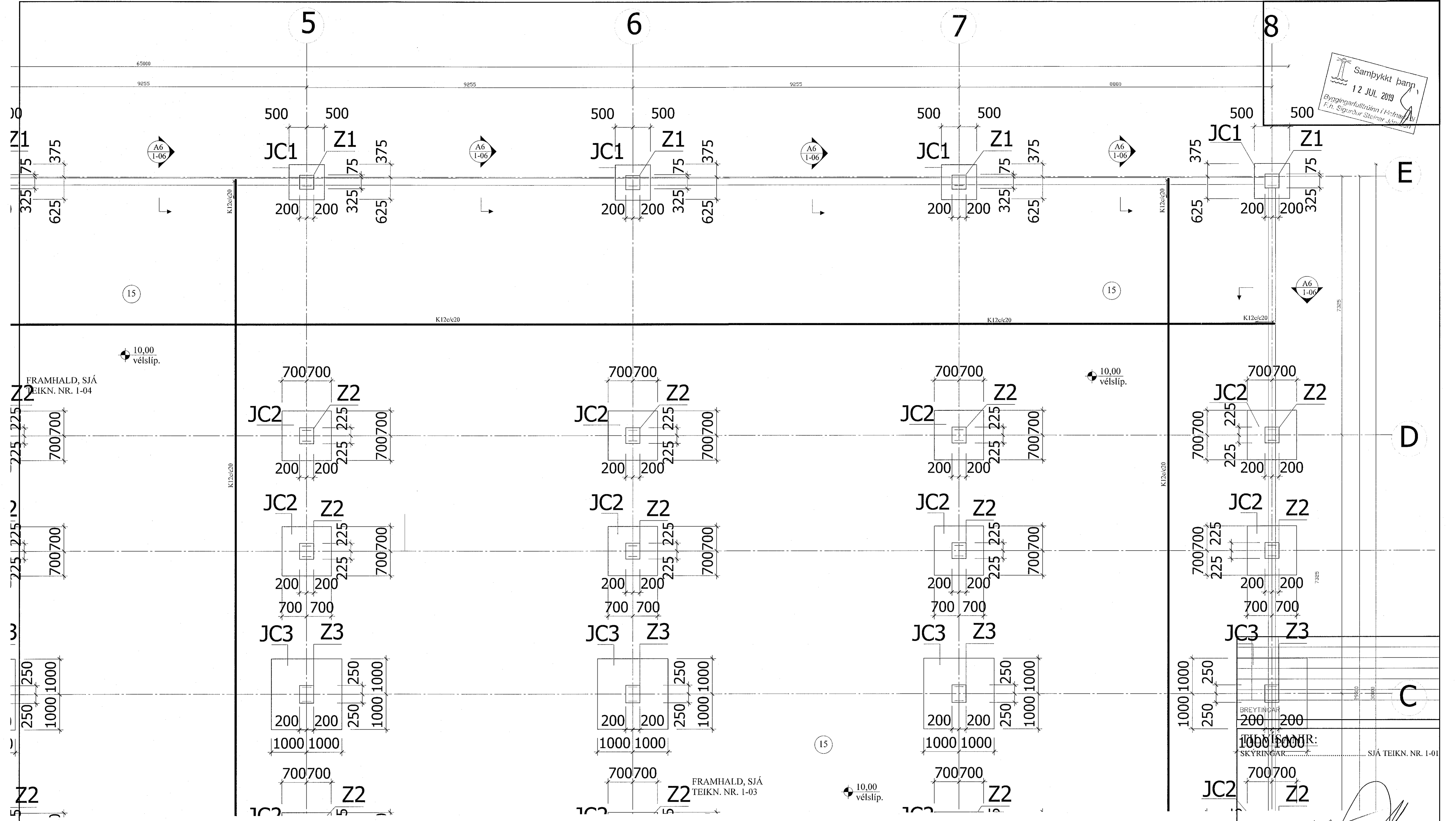
UNDIRSTÖÐUR, GRUNNMYND. 1:50
