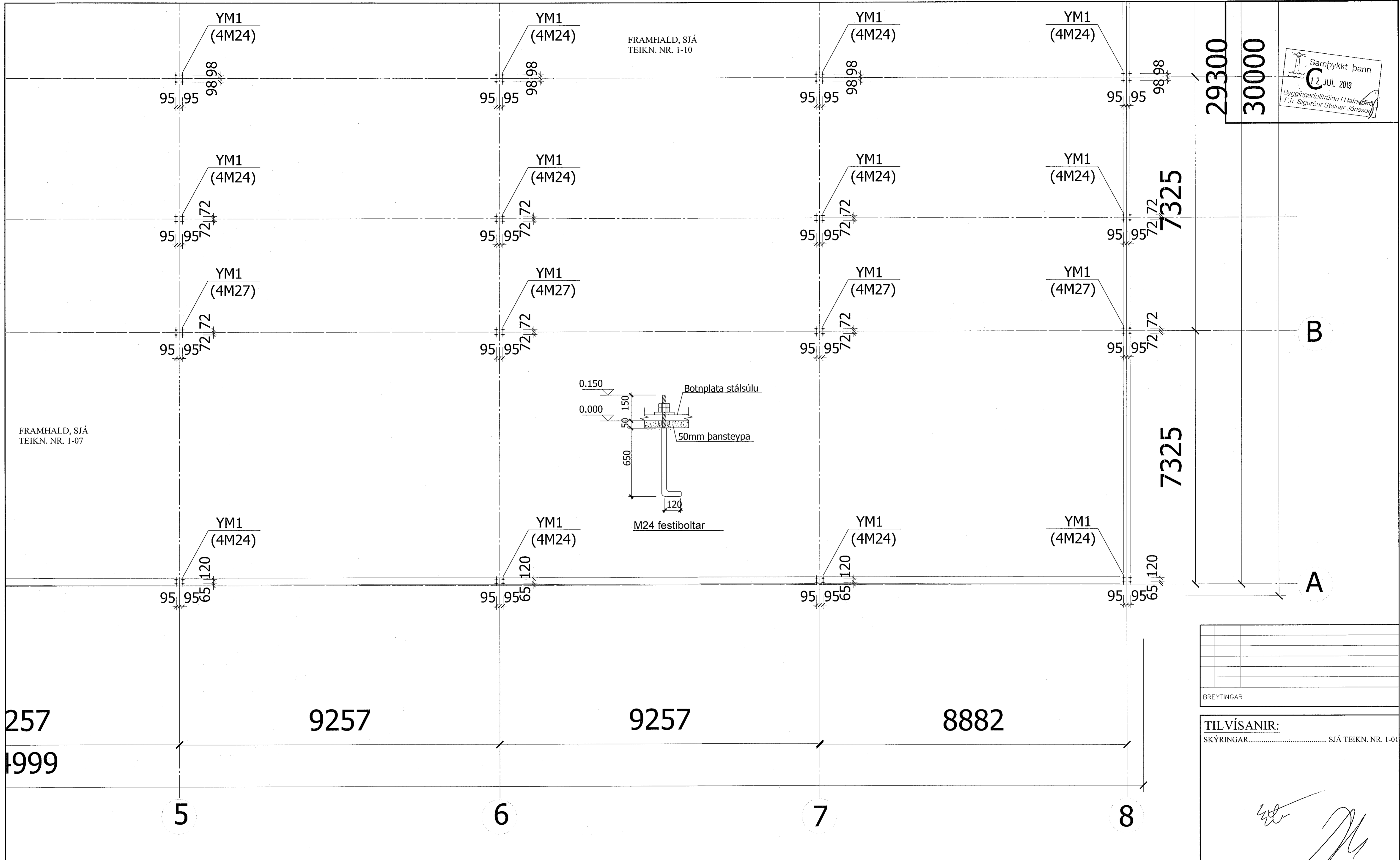
BOLTAÚTSETNING, GRUNNMYND. 1:50
