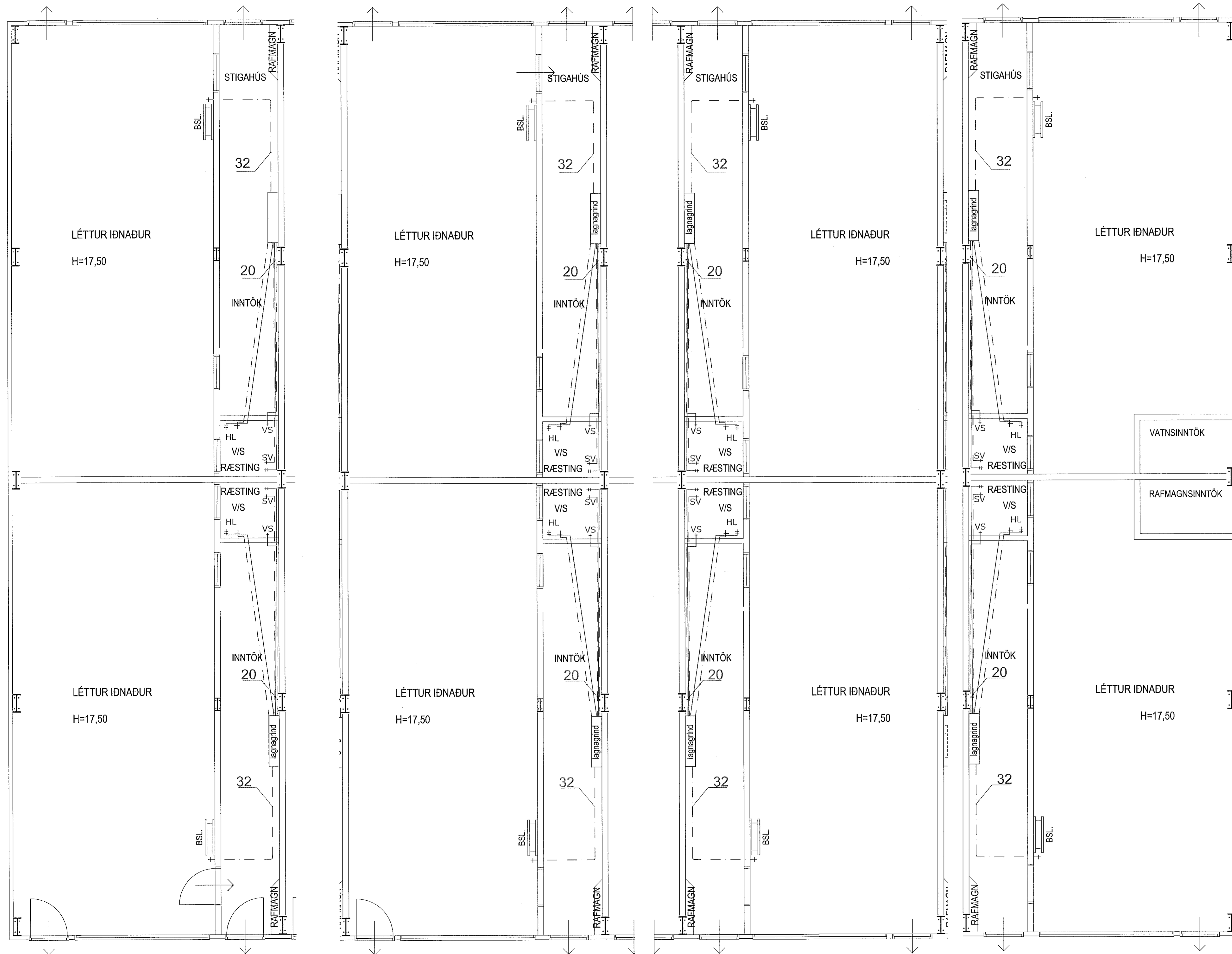
Grunnmynd neysluvatn 1. hæð í hverfi gerð af bilum 1:50
