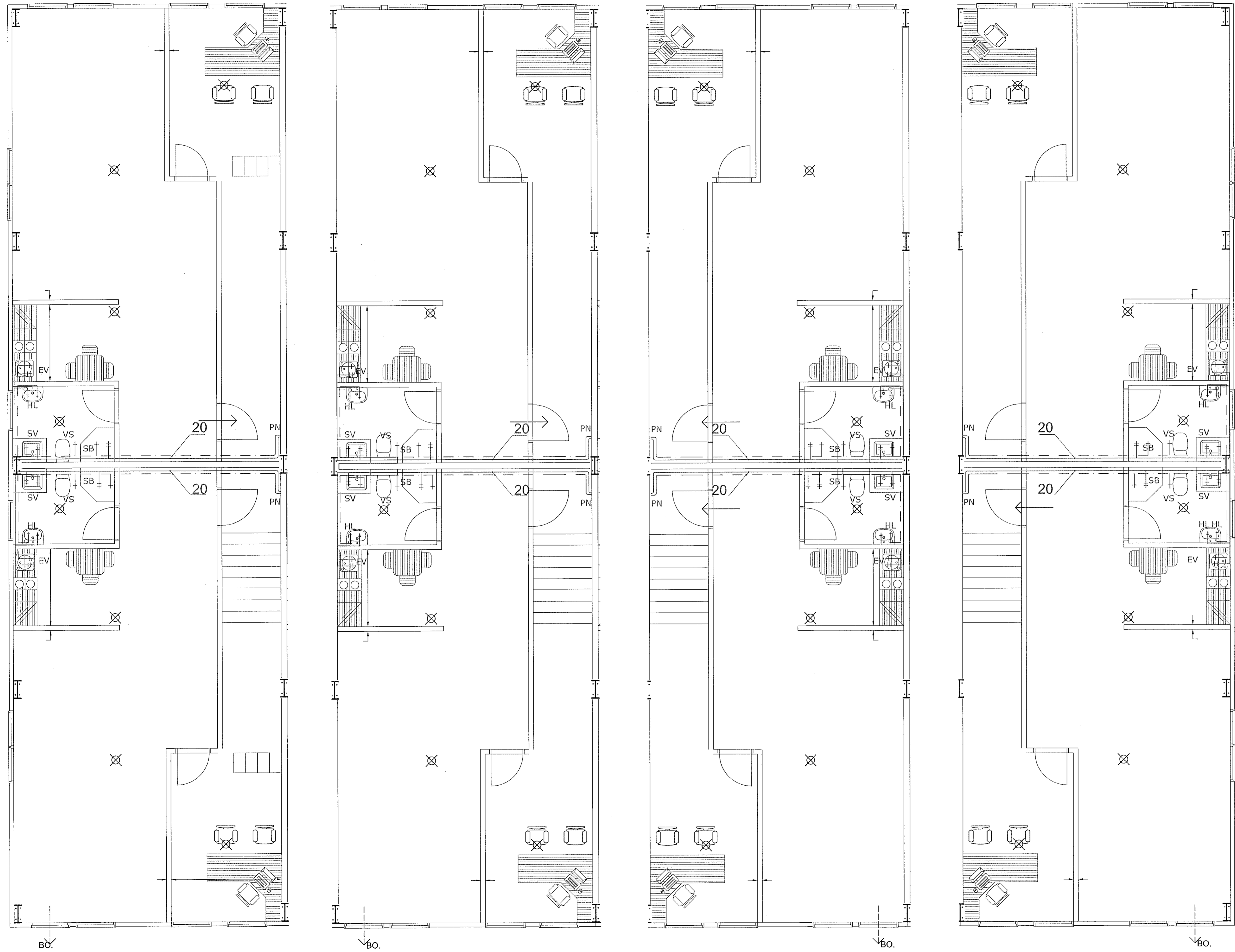
Grunnmynd neysluvatn 2. hæð í hverri gerð af bilum 1:50
