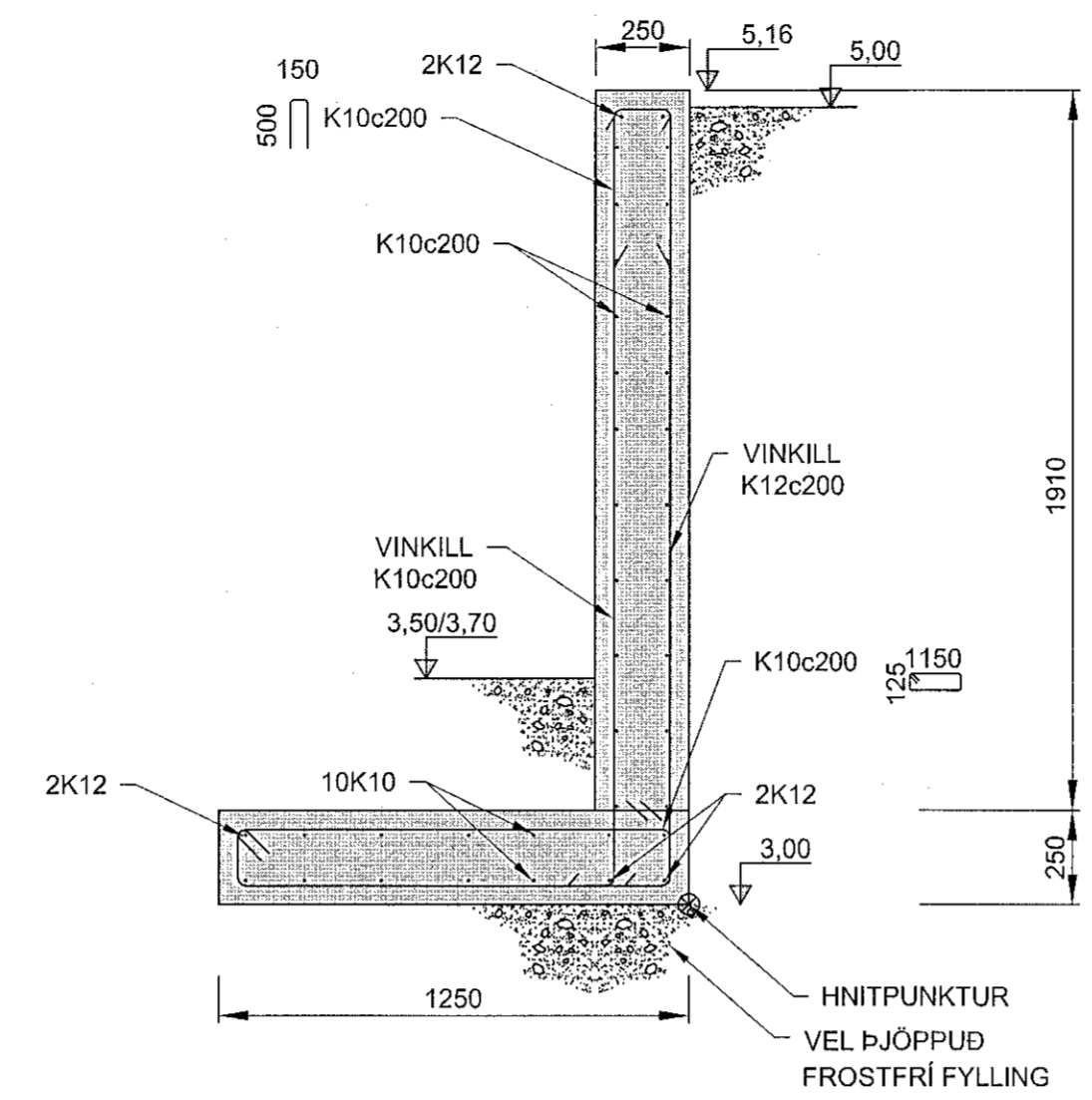
02 SNID (ST02-ST03) 0001 1:20
