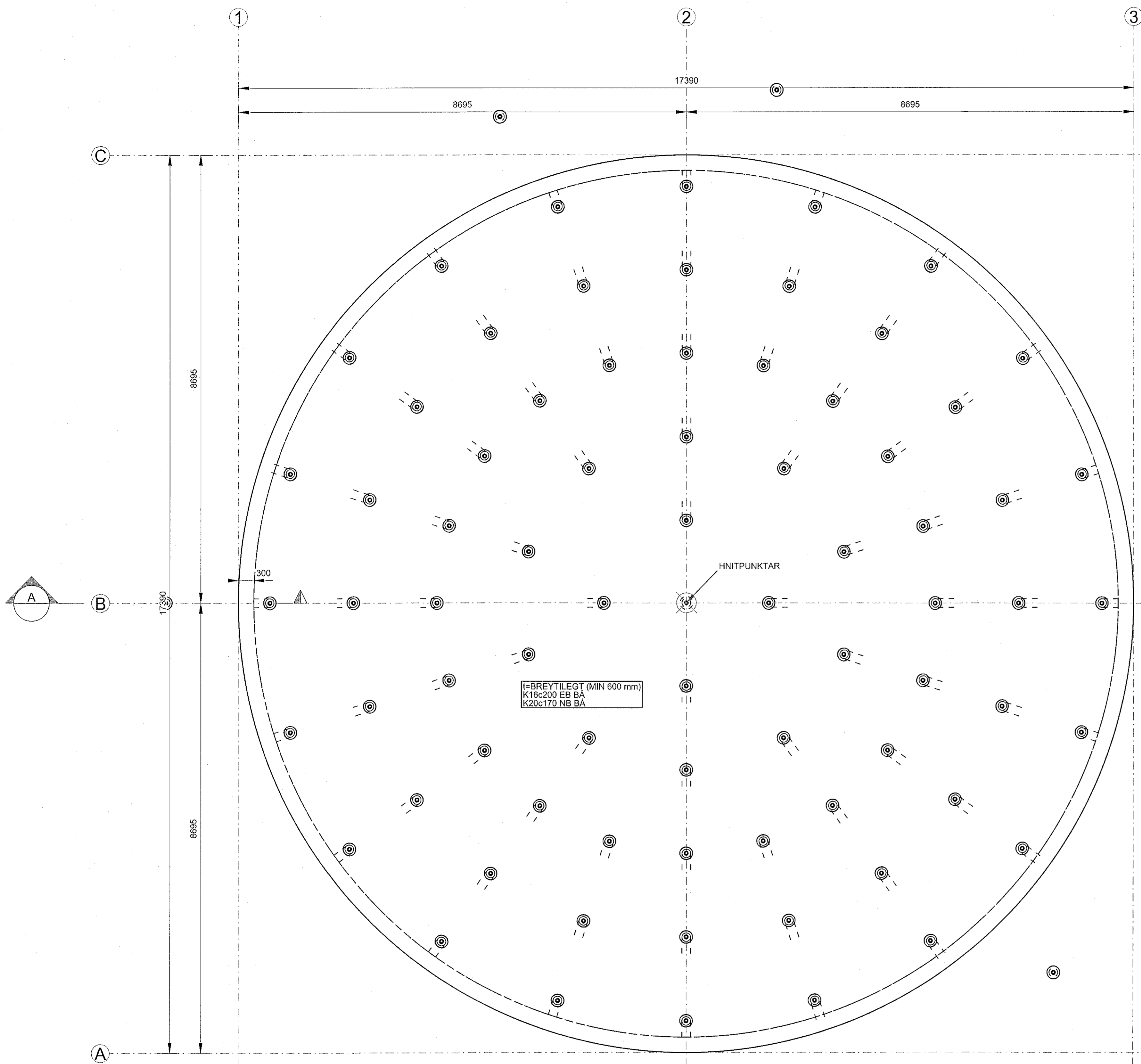
GRUNNMYND 1:50
