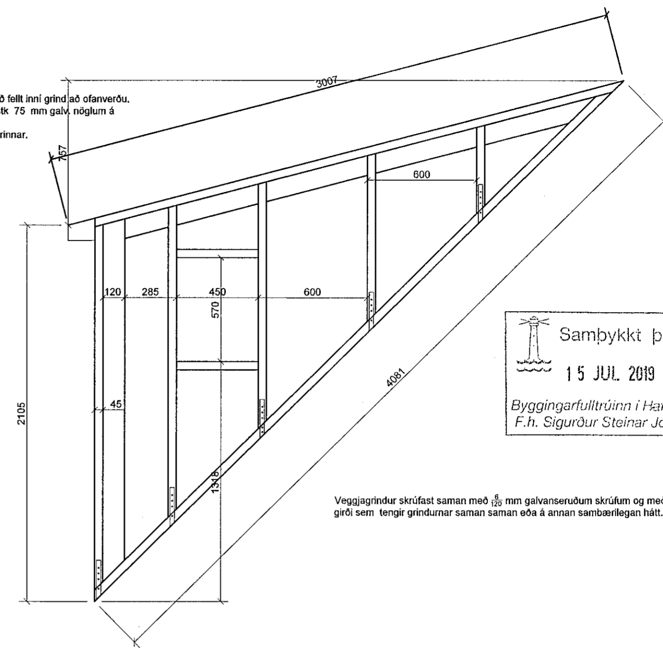
Veggjagrindur hliðar m. 1:50
