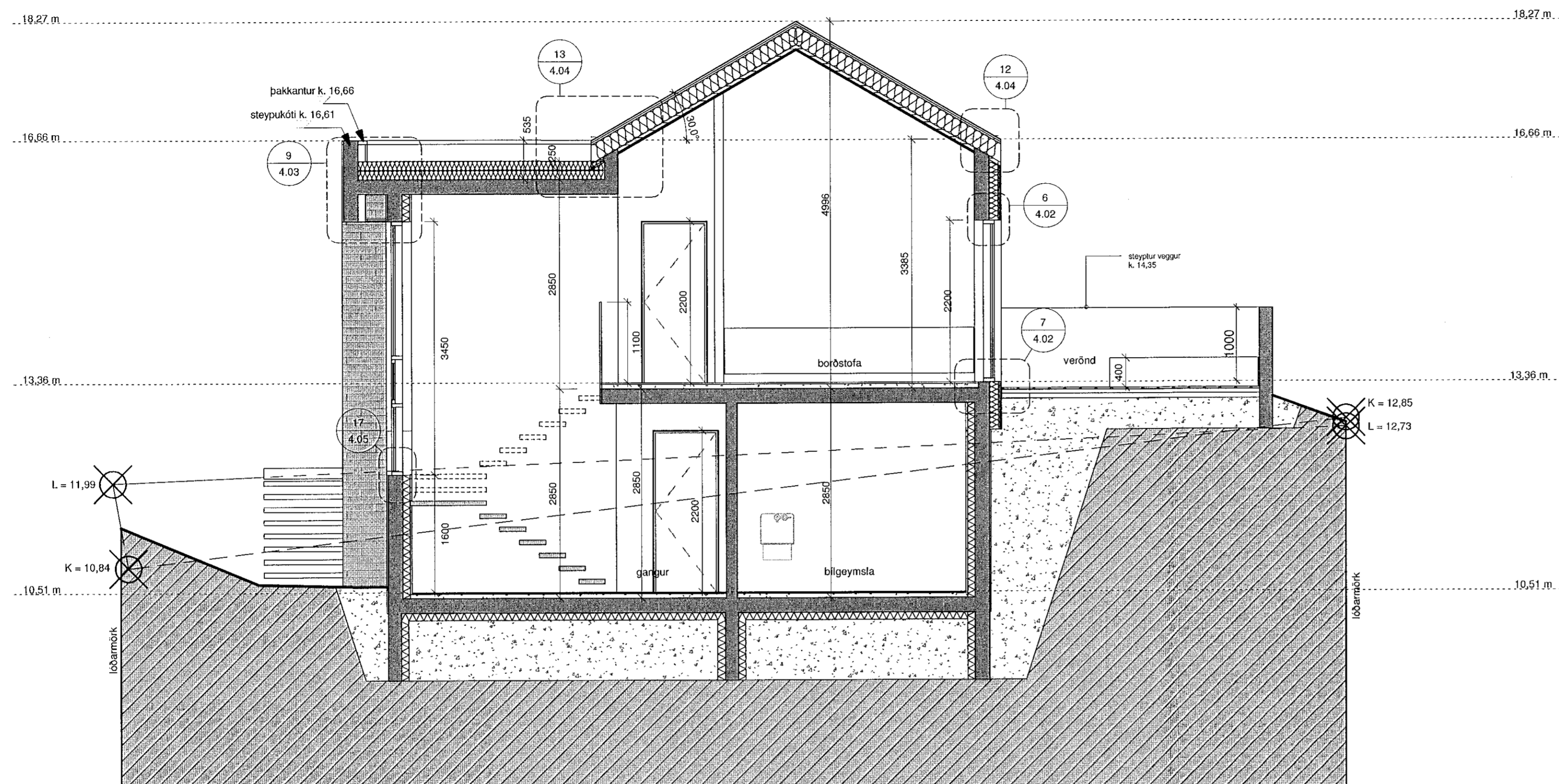
SNEIDING A-A 1:50
