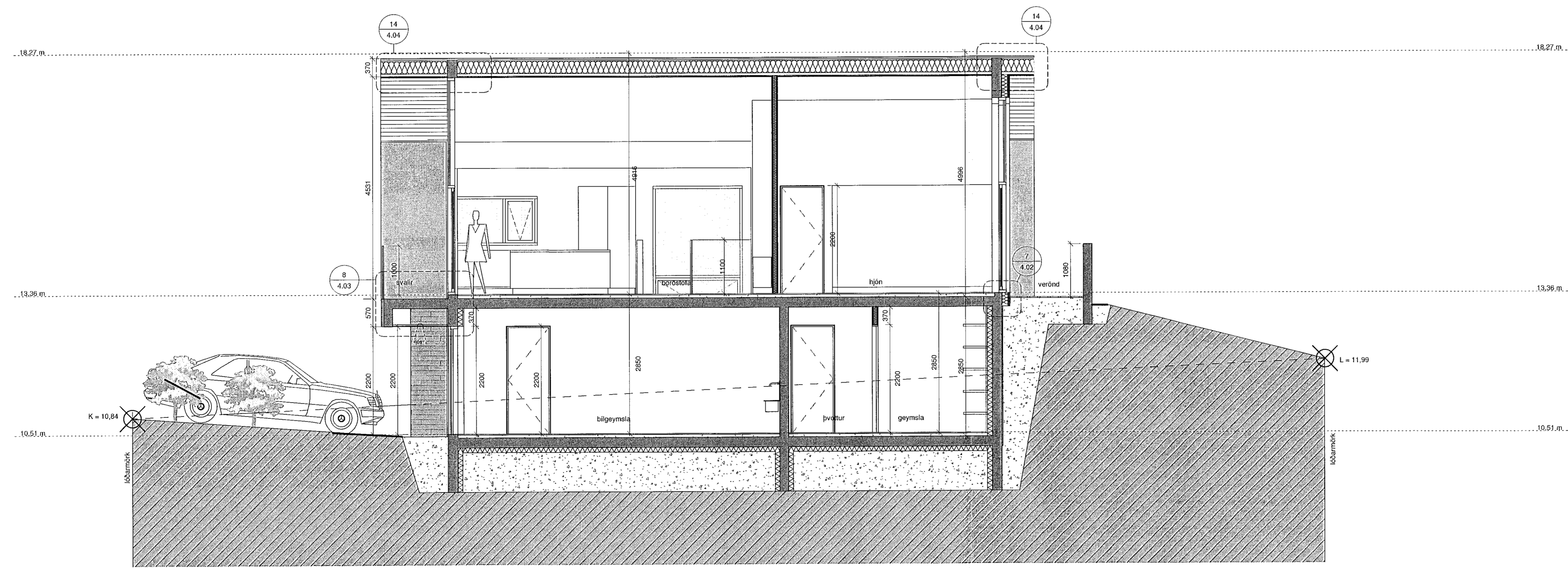
SNEIDING B-B 1:50
