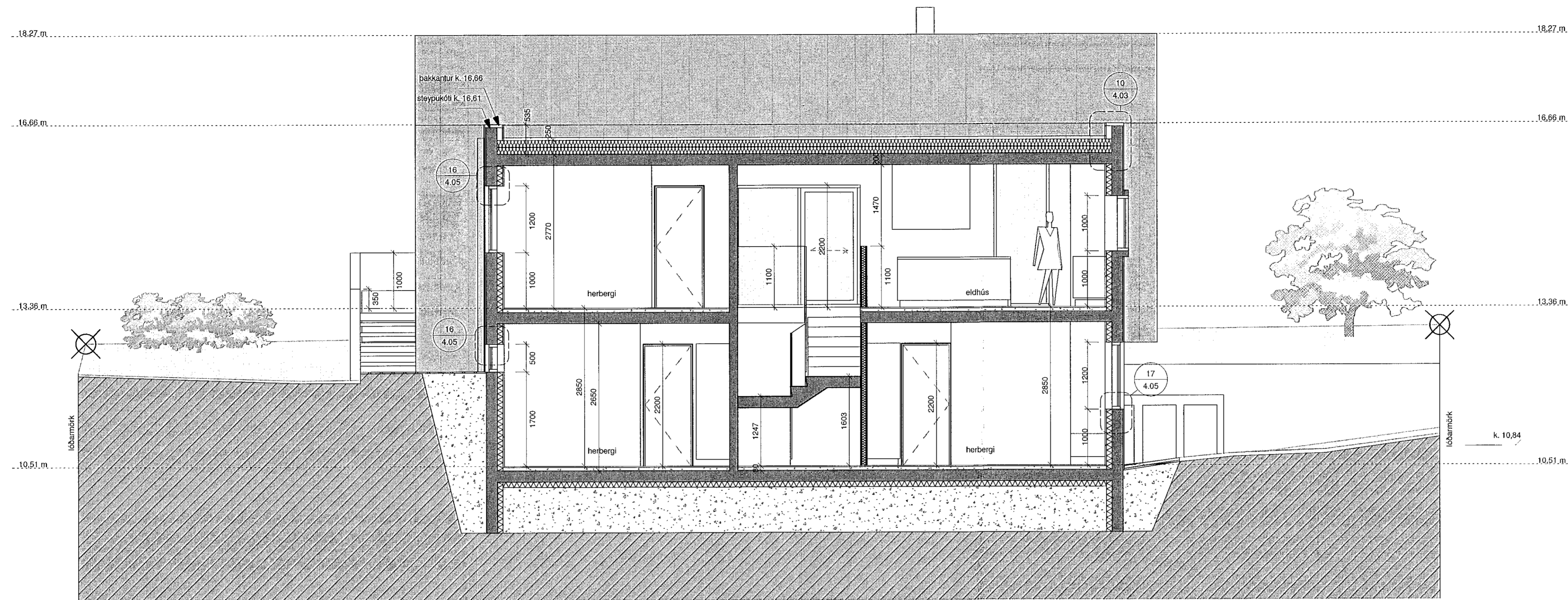
SNEIÐING C-C 1:50
