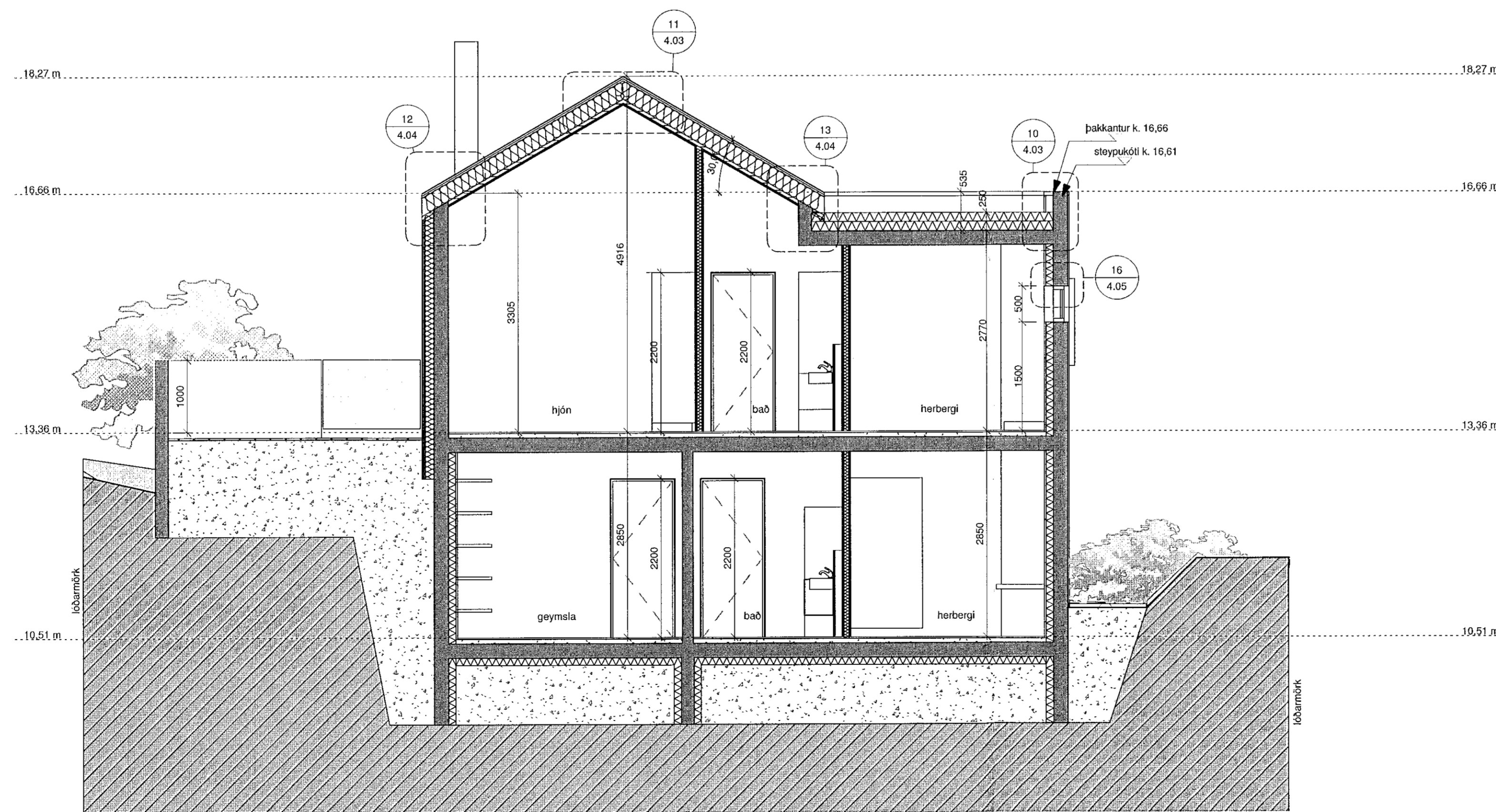
D-D SNEIÐING D-D 1:50
