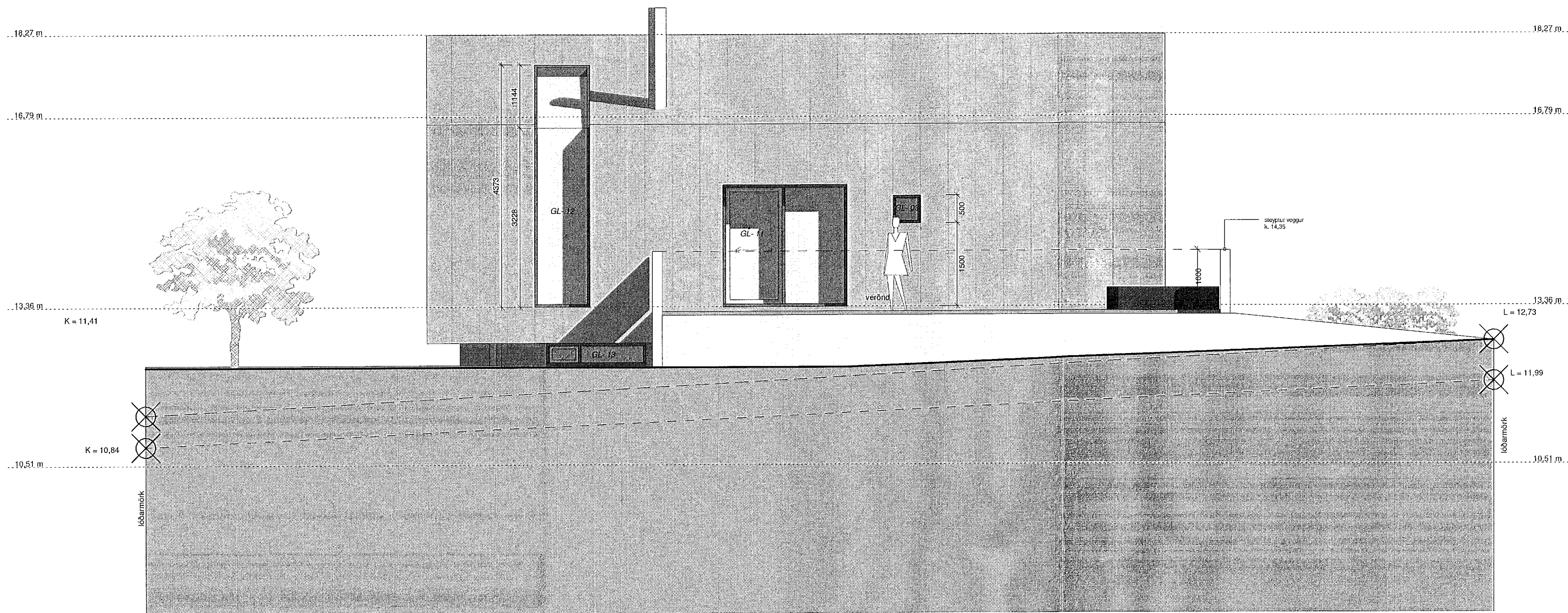
ÚTLIT SUÐVESTUR. 1:50
