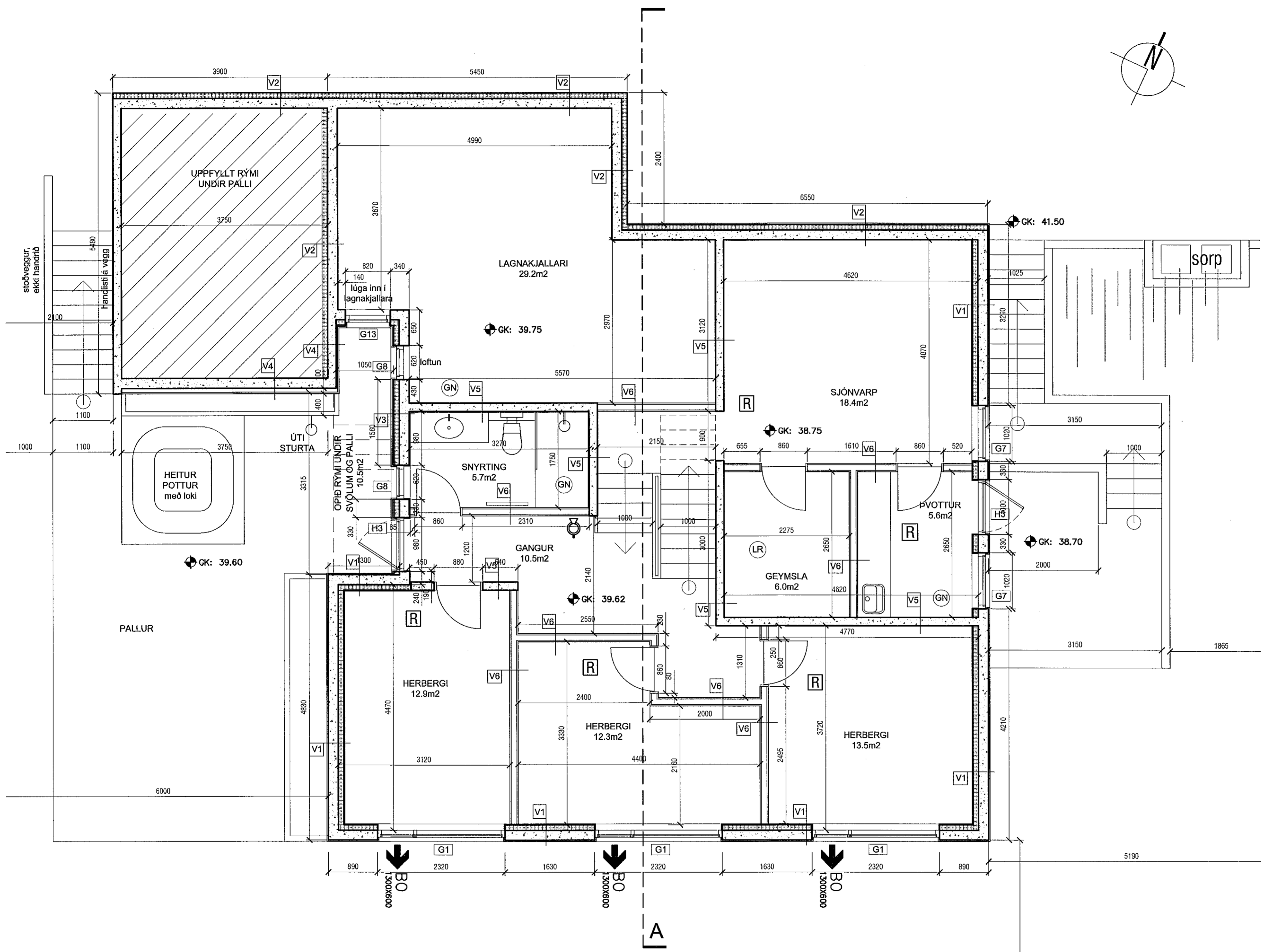
Grunnmynd neðri hæðar mkv. 1:100
