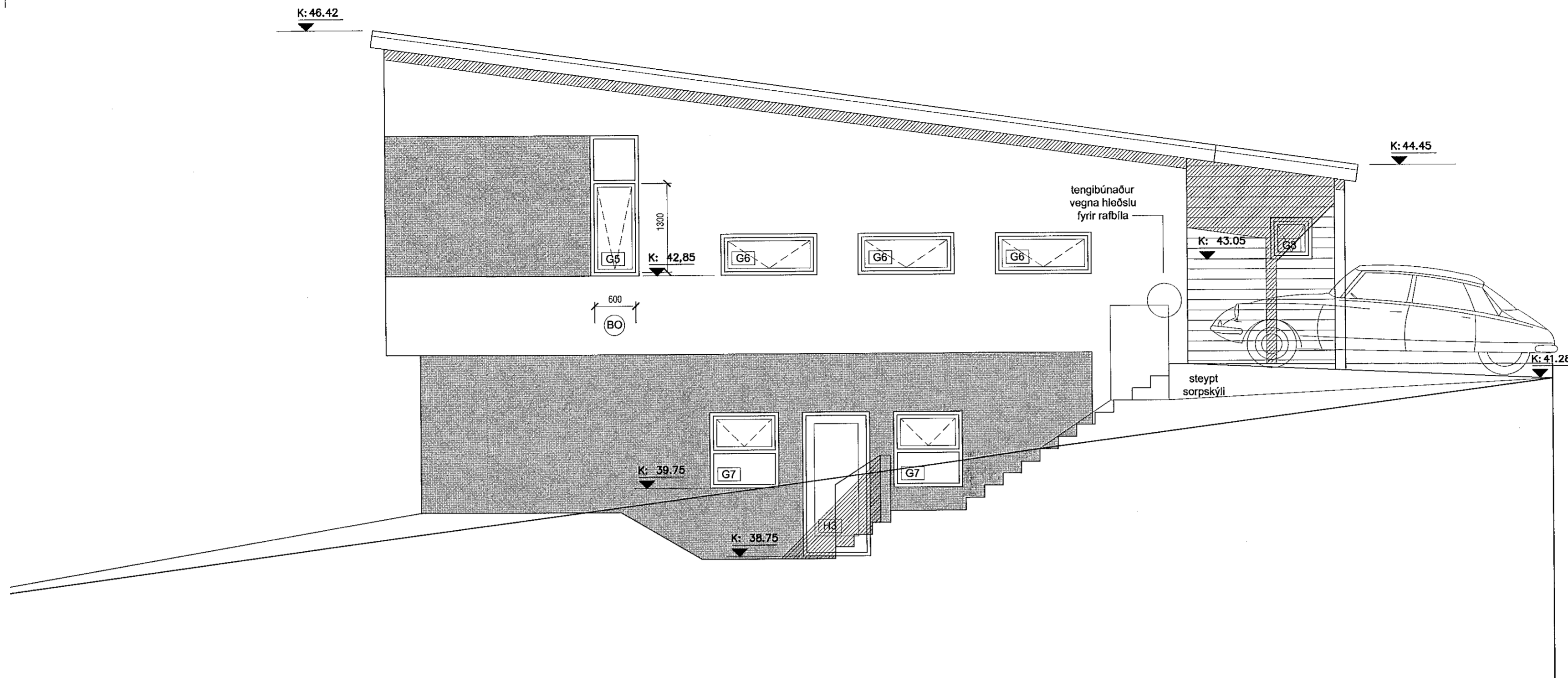
Ásýnd Austur mkv. 1:50
