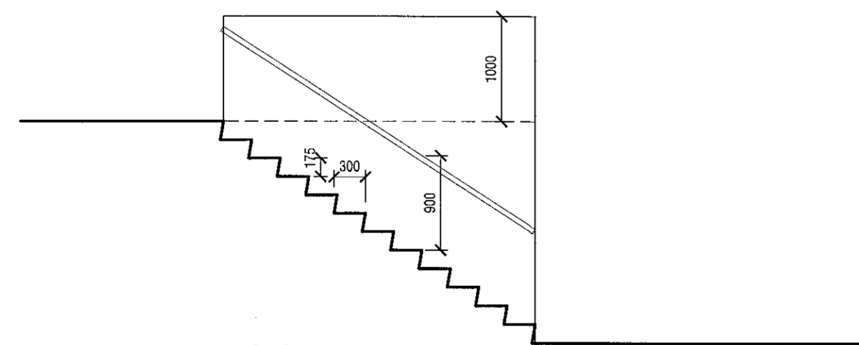
Tröppur á lóð vestur mkv. 1:50
