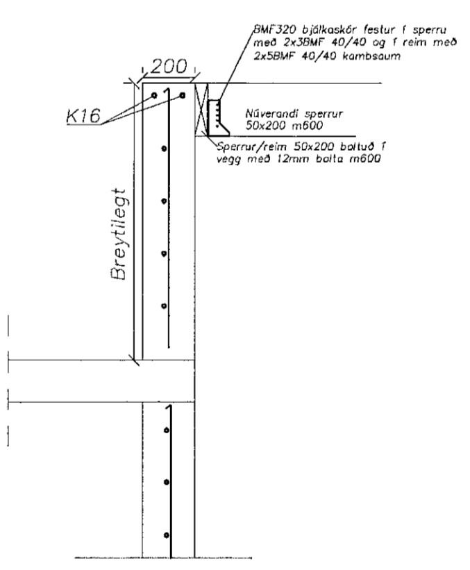
D Snið 1 = 20 mm
