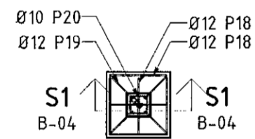
GRUNNMYND SÖKKLA 1 : 50
