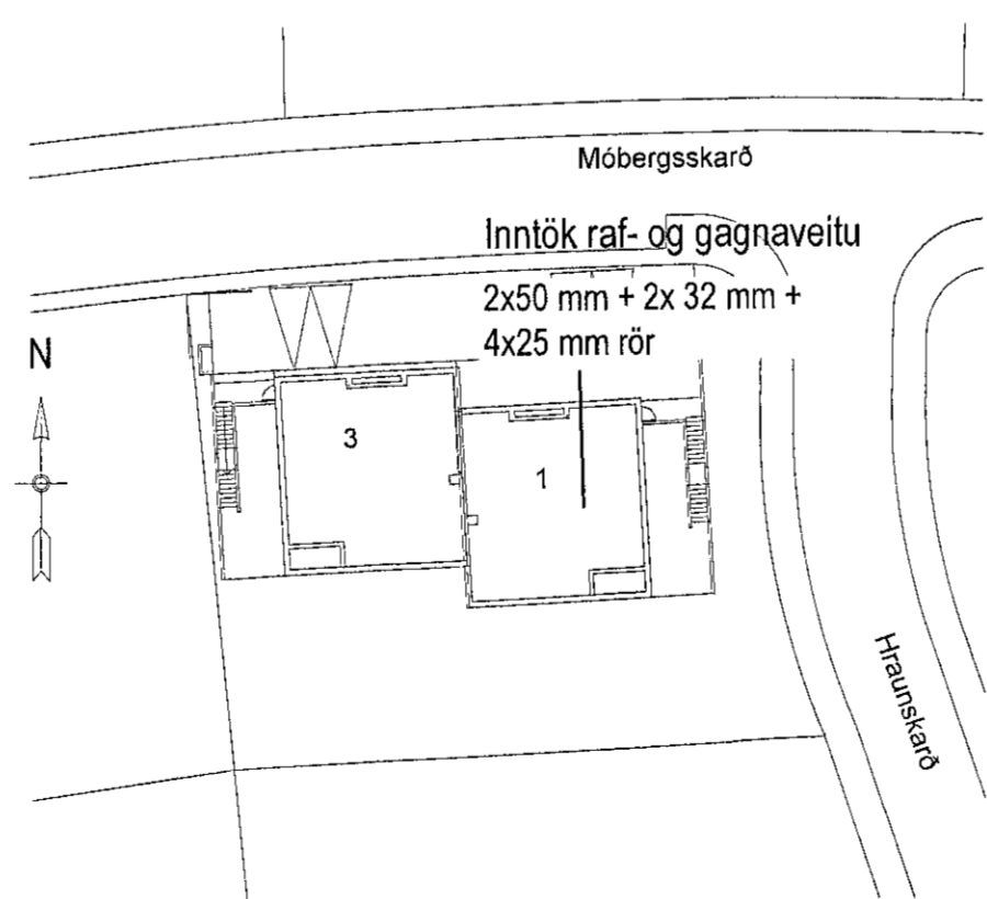
Afstöðumynd Mkv. 1:500
