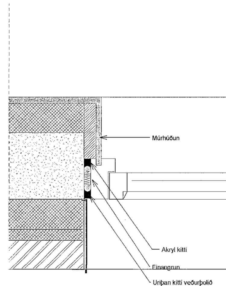
Verkteikn. gluggadeili hlið 1 : 5
