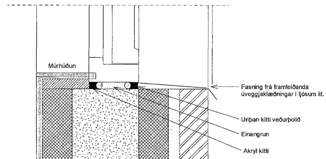
Verkteikn. gluggadeili neðri brún 1 : 5
