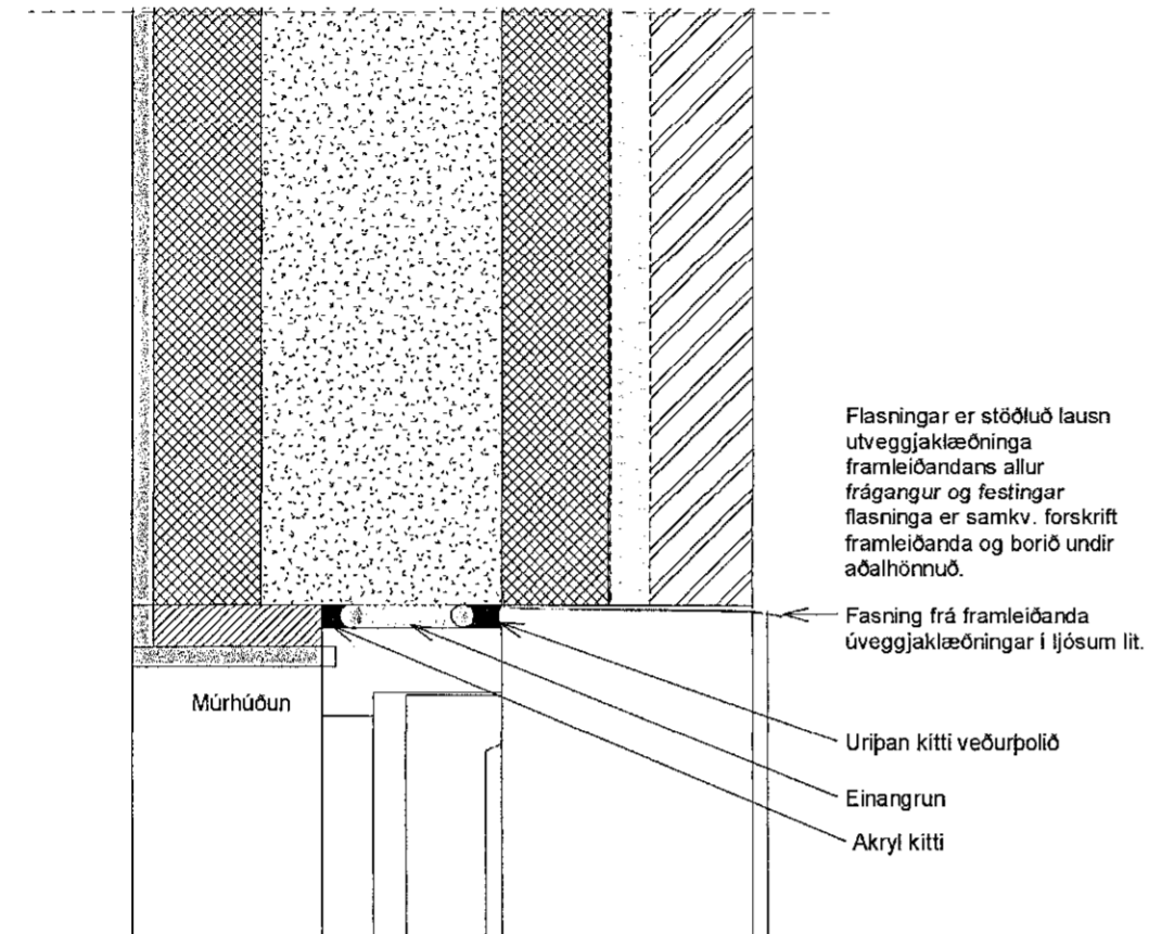
Verkteikn. gluggadeili efri brún 1 : 5
