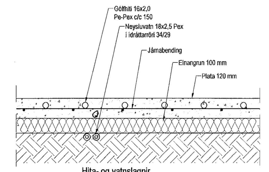
Hita- og vatnslagnir, Snið í botnþlöt, 1:10
