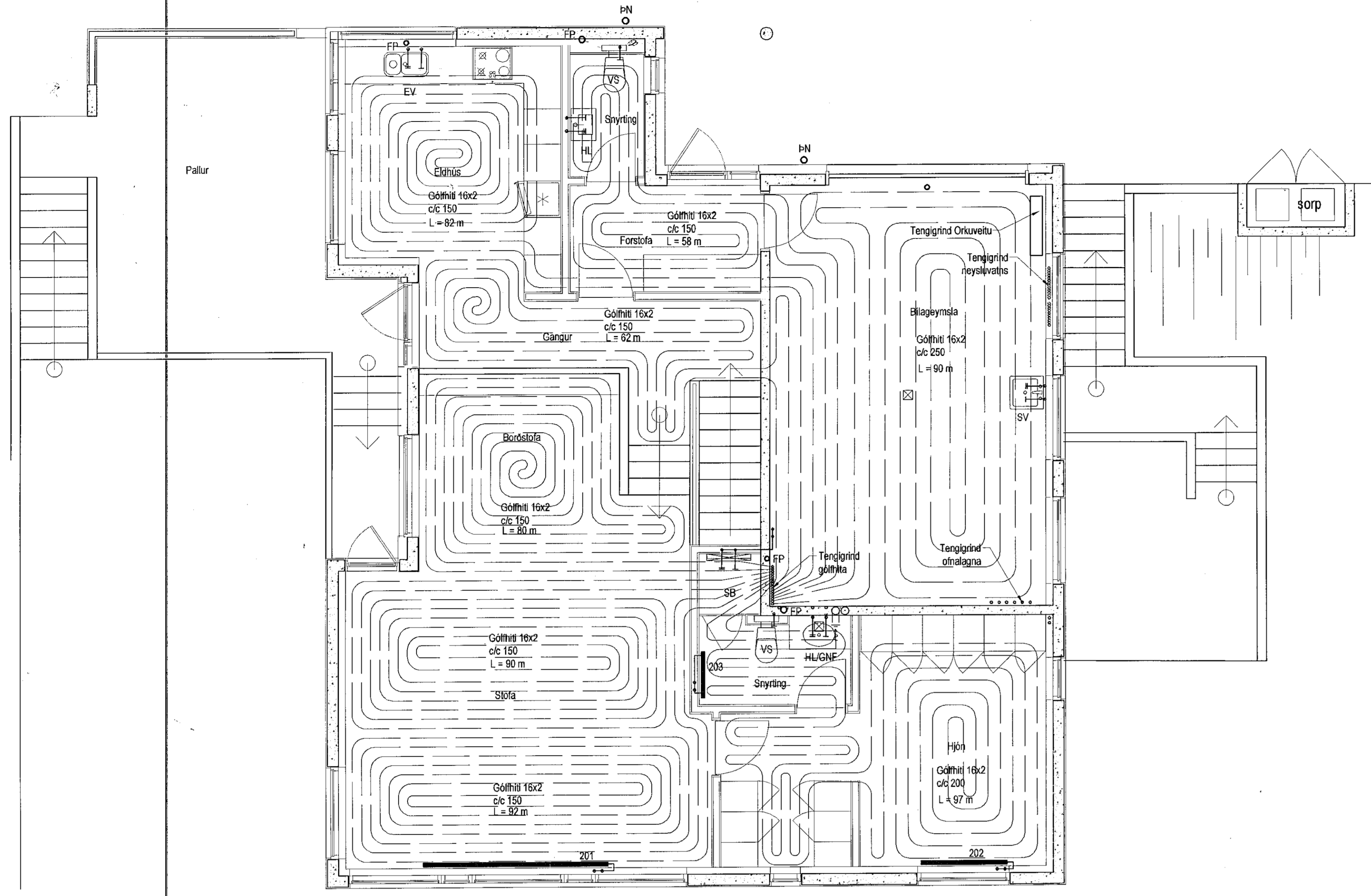
Gólfhitalagnir 2. hæð, 1:50
