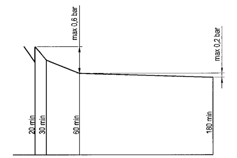
Þrýstiprófan á neysluvatnslögnum línurit
