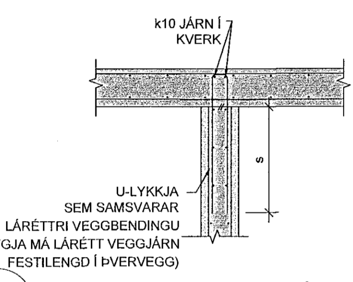
K4 LÄRÉTT KENNISNIÐ - VEGGMÓT Mkv. 2
