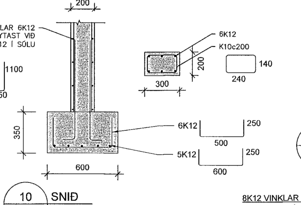
U1 UNDIRSTADA U1 Mkv. 2
