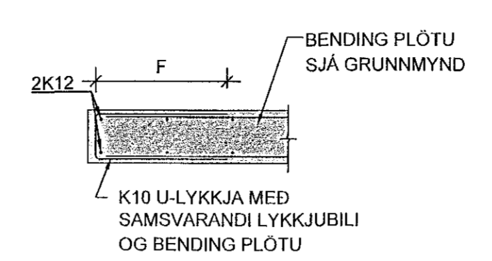
K2 LÖÐRÉTT KENNISNIÐ - PLÖTUBRÚN Mkv. 2
