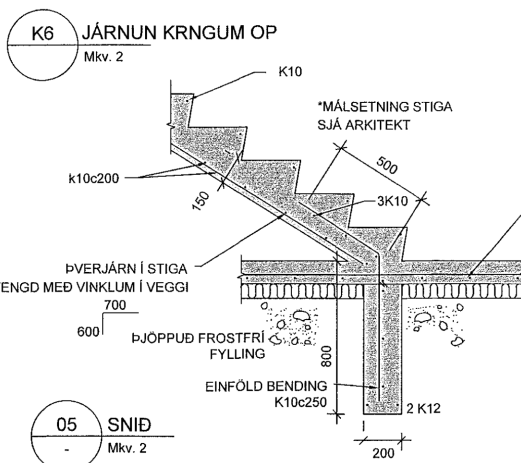
K6 JÄRNUN KRINGUM OP Mkv. 2
