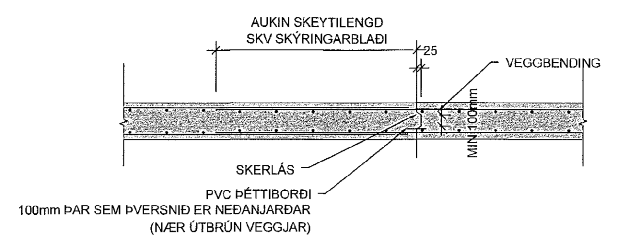
K1 LÄRÉTT KENNISNIÐ - SKERLÄS Í 200/250mm VEGG Mkv. 2
