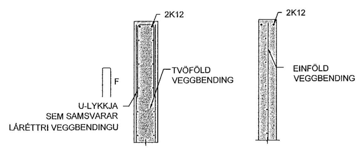
K5 LÄRÉTT KENNISNIÐ - VEGGENDI TVÖFÖLD BENDING OG EINFÖLD VEGGBENDING Mkv. 2
