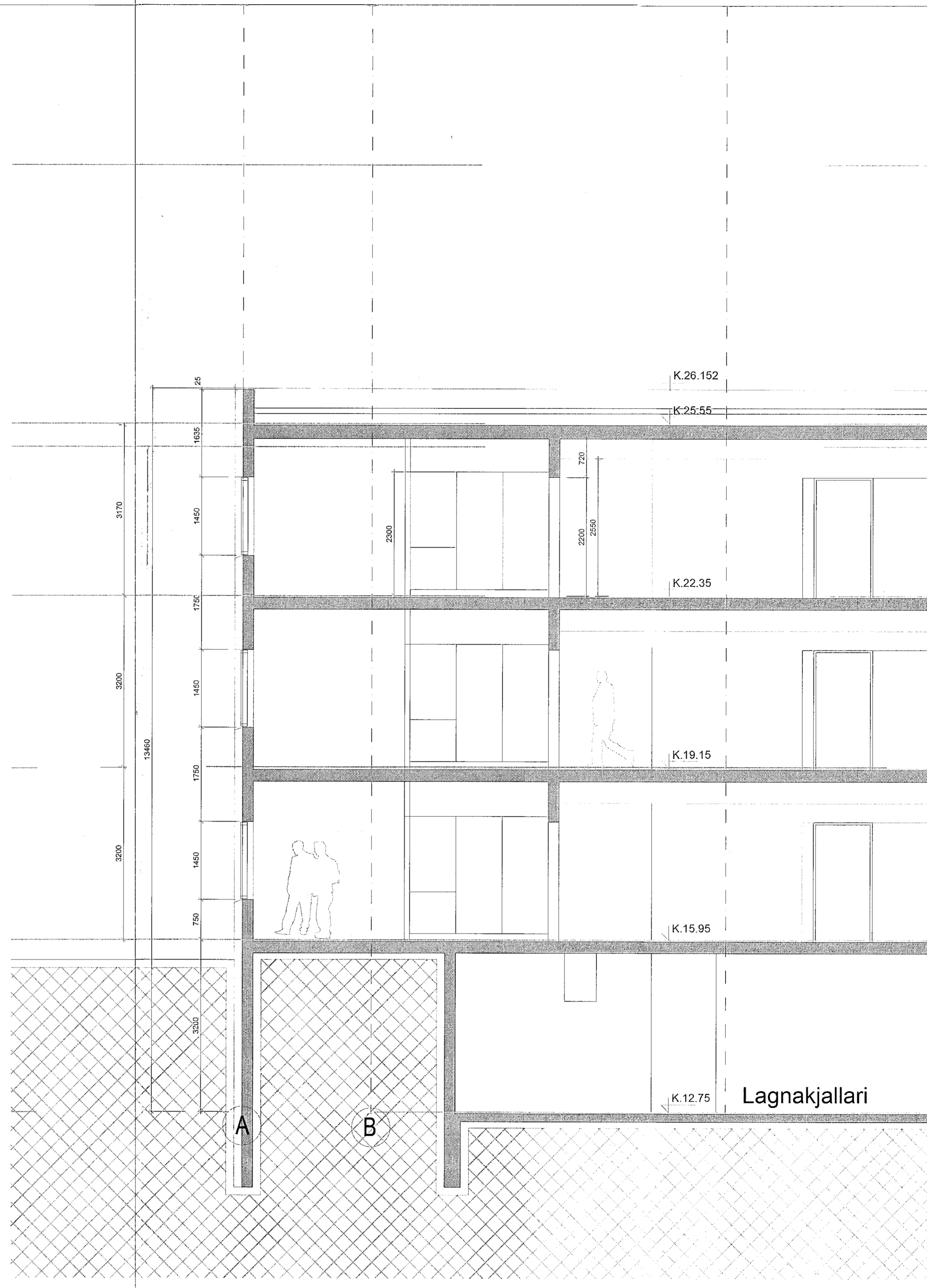
SNID A-A 1:50
