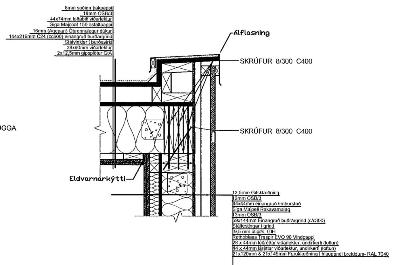
TENING ÞAKS OG ÚTVEGGJAR, KENNISNIÐ, 1:10
