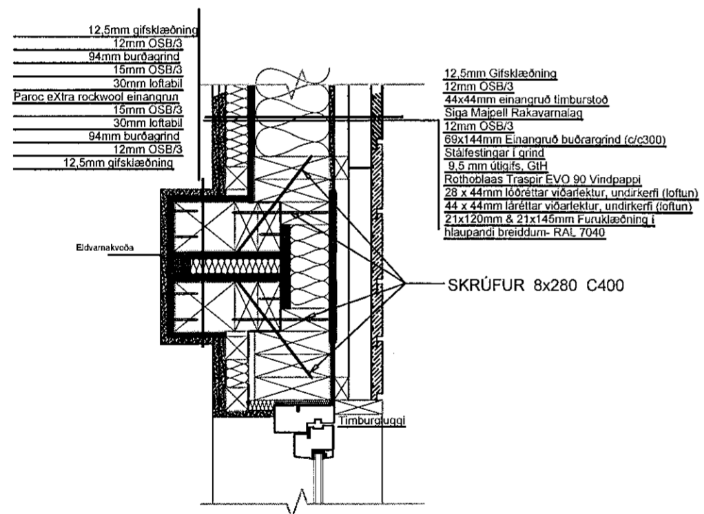
TENING TVEGGJA EINGA, KENNISNIÐ, 1:10
