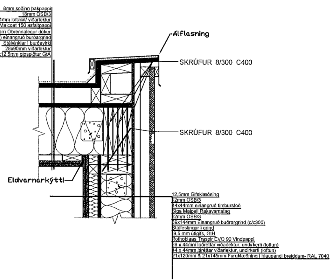
TENING ÞAKS OG ÚTVEGGJAR, KENNISNIÐ, 1:10
