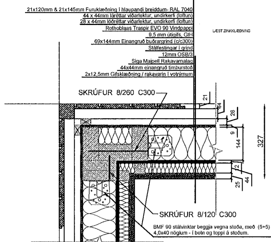
FRÁGANGUR Á ÚTHORNI, KENNISNIÐ, 1:10
