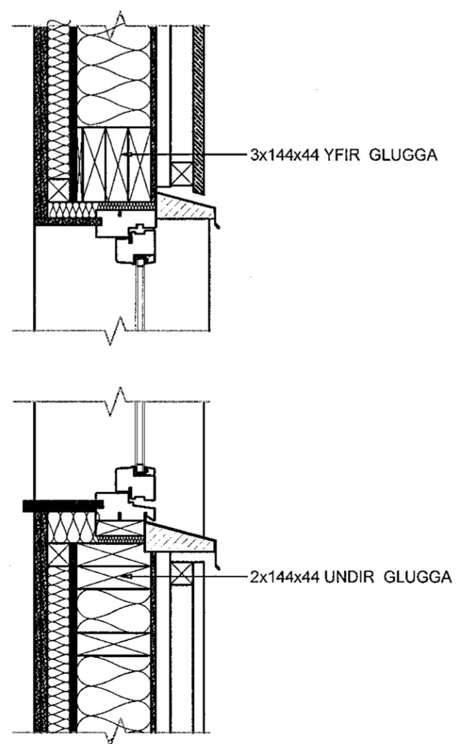
FRÁGANGUR YFIR OG UNDIR GLUGGA, KENNISNIÐ, 1:10
