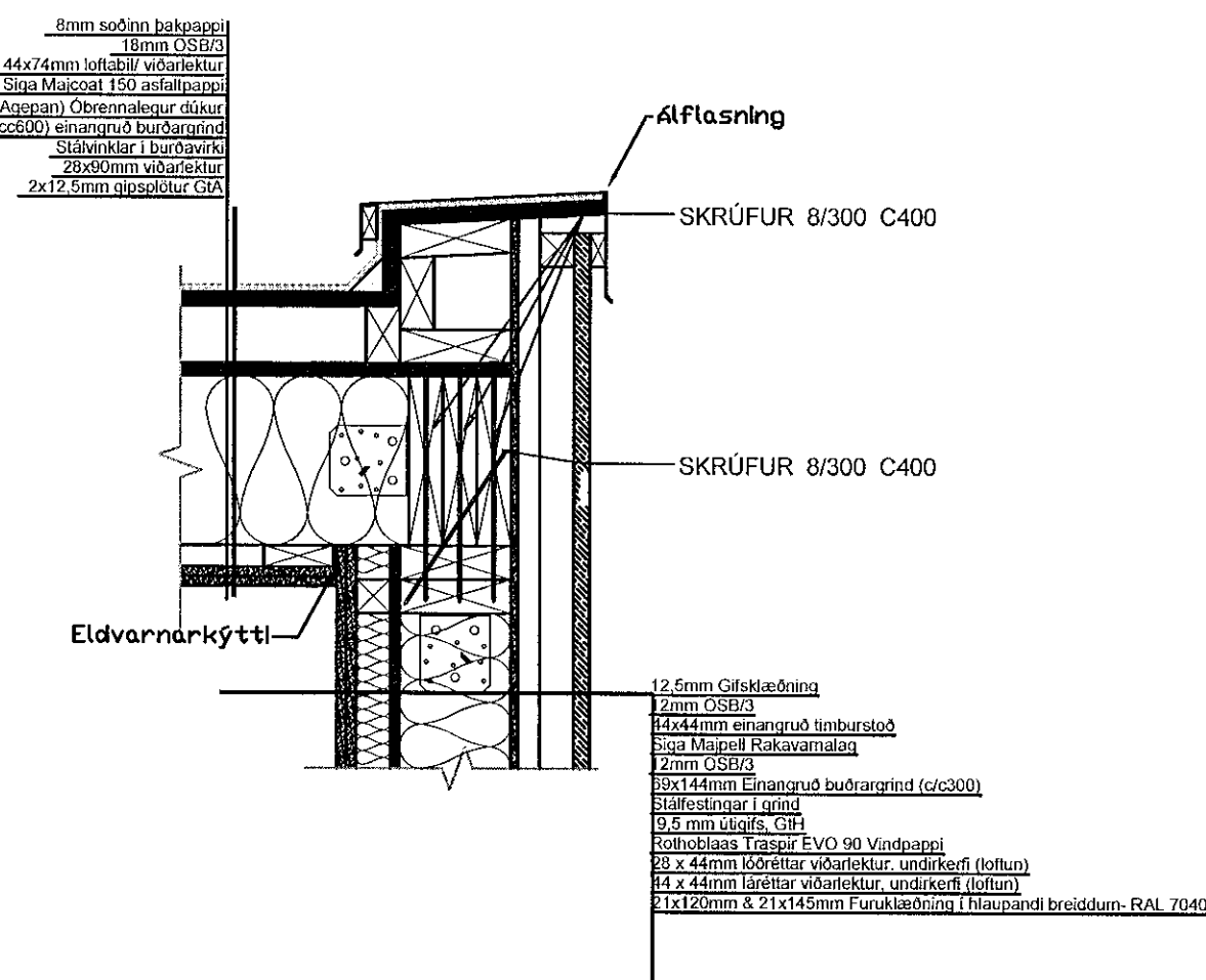
TENING ÞAKS OG ÚTVEGGJAR, KENNISNIÐ, 1:10
