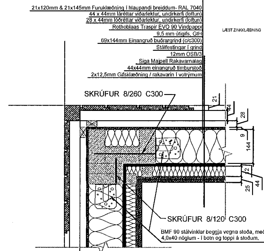
FRÁGANGUR Á ÚTHORNI, KENNISNIÐ, 1:10
