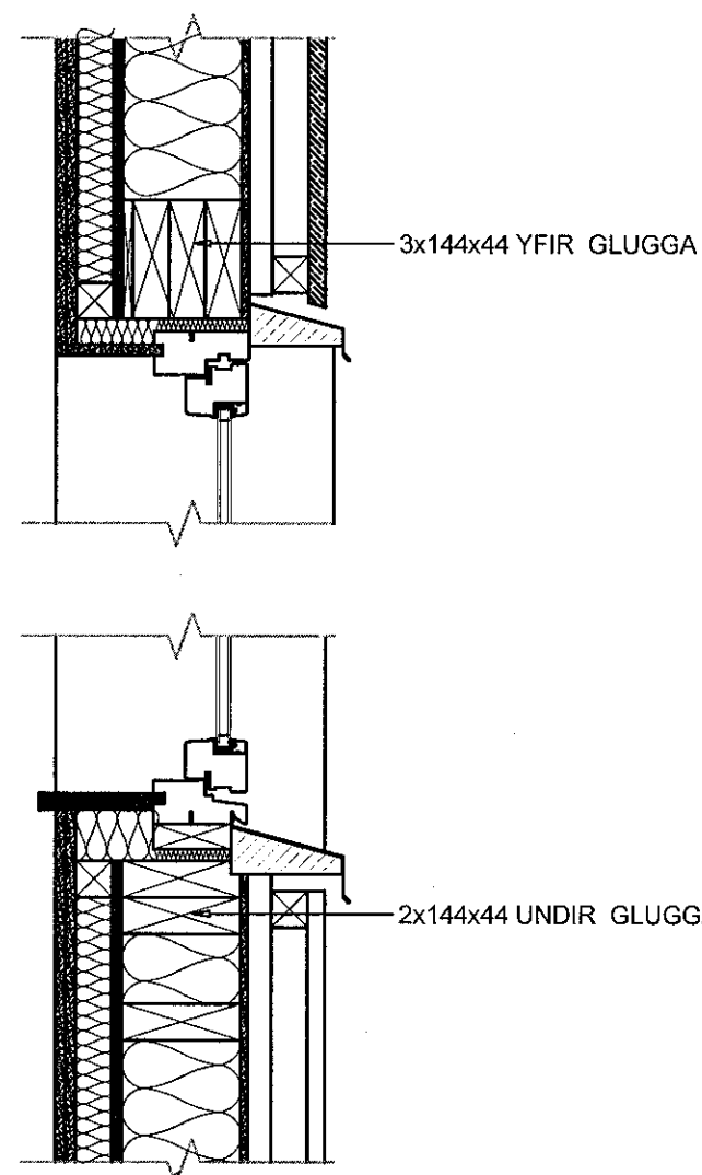
FRÁGANGUR YFIR OG UNDIR GLUGGA, KENNISNIÐ, 1:10
