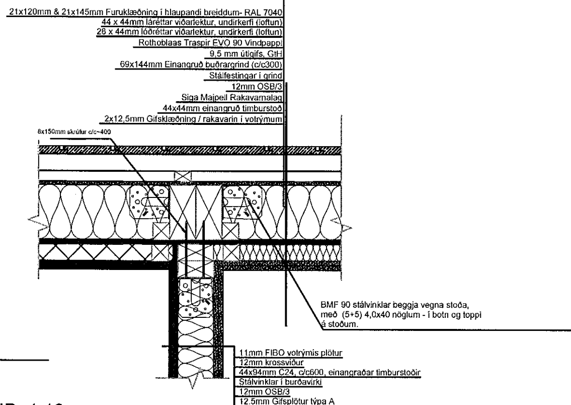
TENING INN- OG ÚTVEGGJAR, KENNISNIÐ, 1:10
