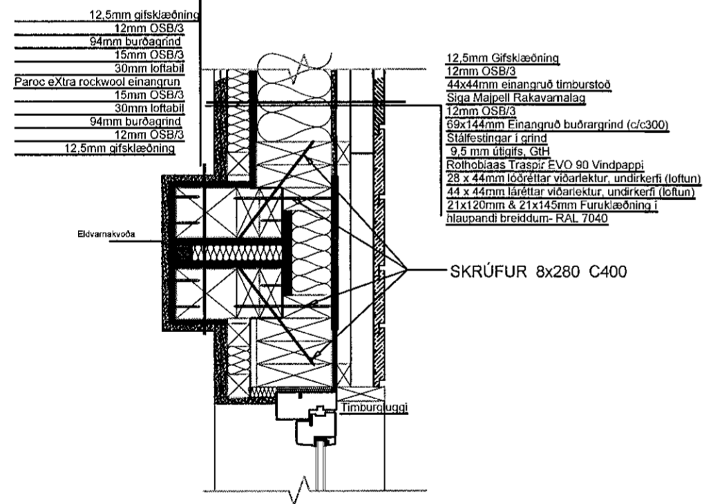
TENNING TVEGGJA EINGA, KENNISNIÐ, 1:10
