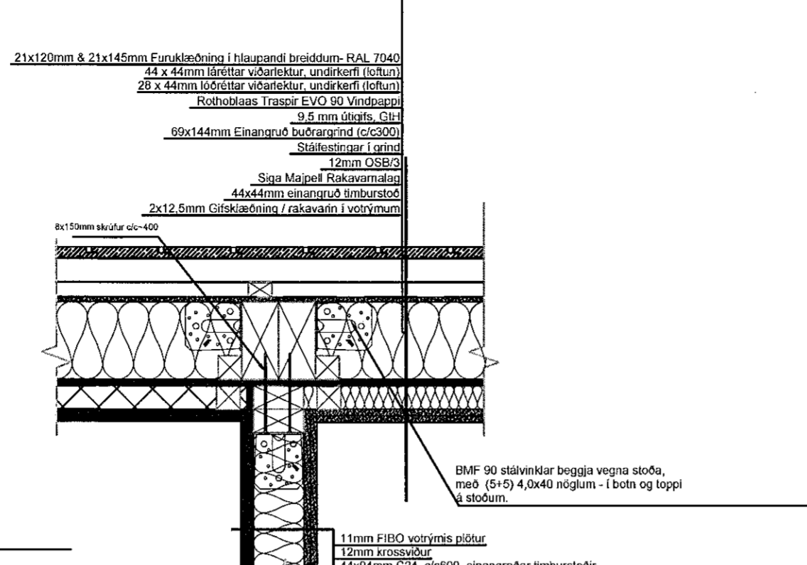
TENNING INN- OG ÚTVEGGJAR, KENNISNIÐ, 1:10
