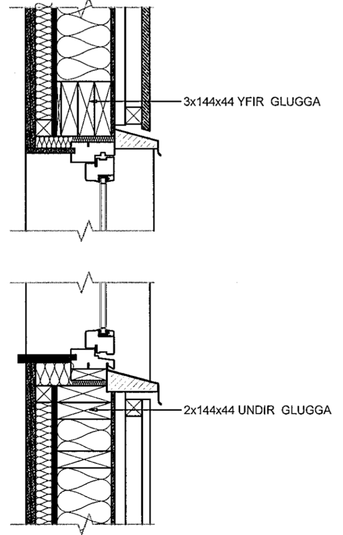
FRÁGANÐUR YFIR OG UNDIR GLUGGA, KENNISNIÐ, 1:10
