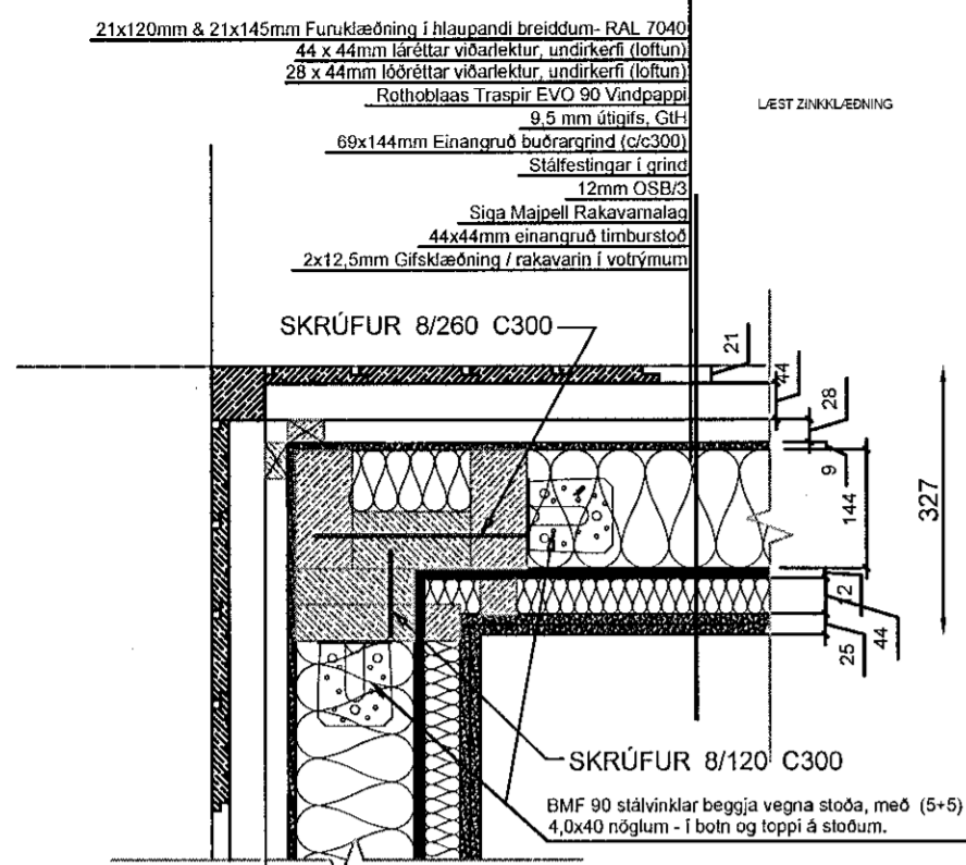
FRÁGANÐUR Á ÚTHORNI, KENNISNIÐ, 1:10
