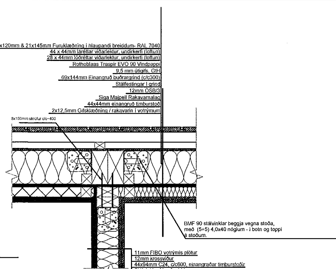
TENING INN- OG ÚTVEGGJAR, KENNISNIÐ, 1:10
