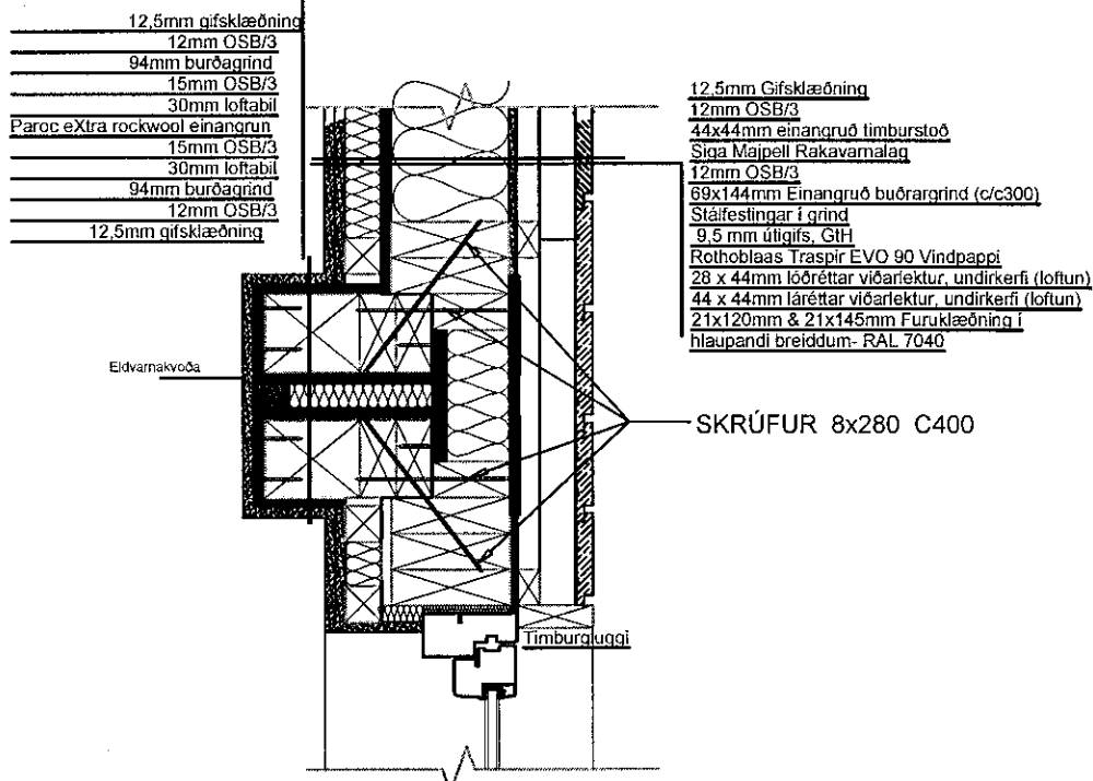
TENING TVEGGJA EINGA, KENNISNIÐ, 1:10
