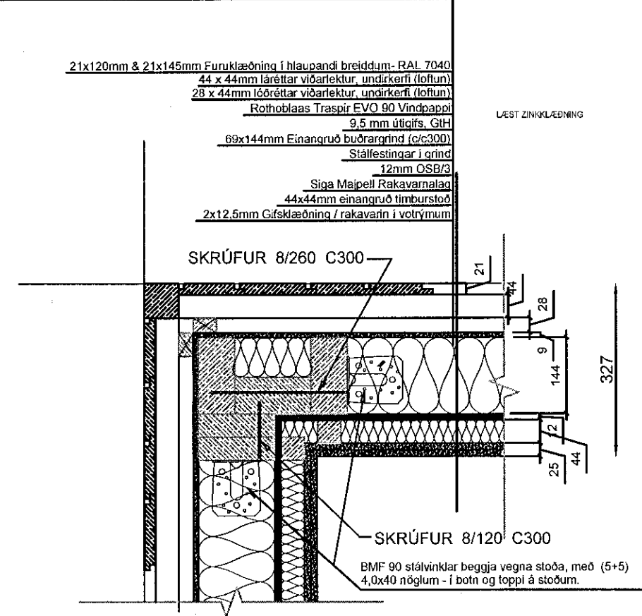
FRÁGANGUR Á ÚTHORNI, KENNISNIÐ, 1:10
