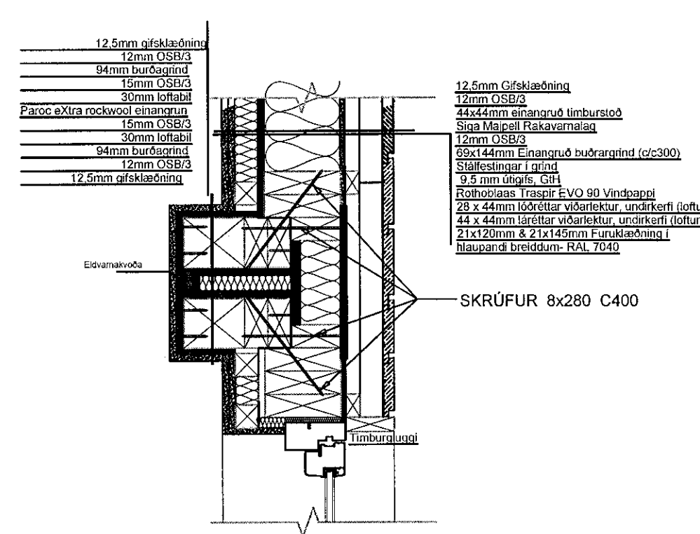
TENING TVEGGJA EINGA, KENNISNIÐ, 1:10
