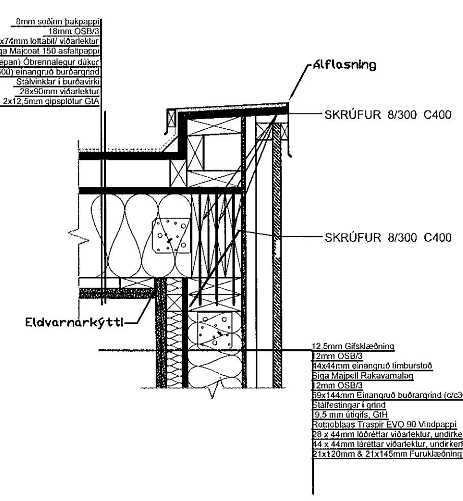
TENING ÞAKS OG ÚTVEGGJAR, KENNISNIÐ, 1:10
