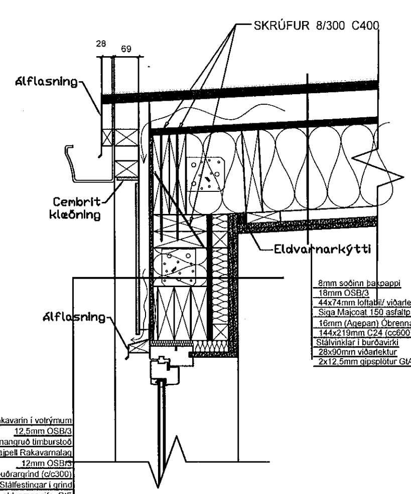
TENING ÞAKS OG ÚTVEGGJAR, KENNISNIÐ, 1:10
