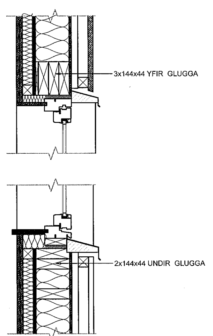
FRÁANGUR YFIR OG UNDIR GLUGGA, KENNISNIÐ, 1:10
