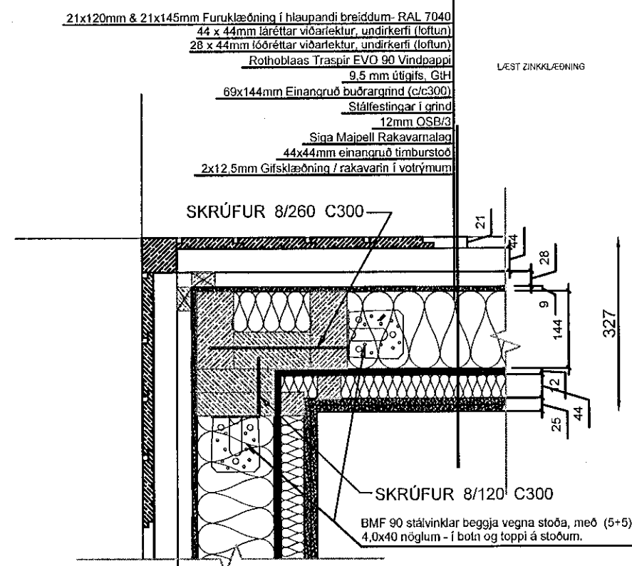
FRÁANGUR Á ÚTHORNI, KENNISNIÐ, 1:10
