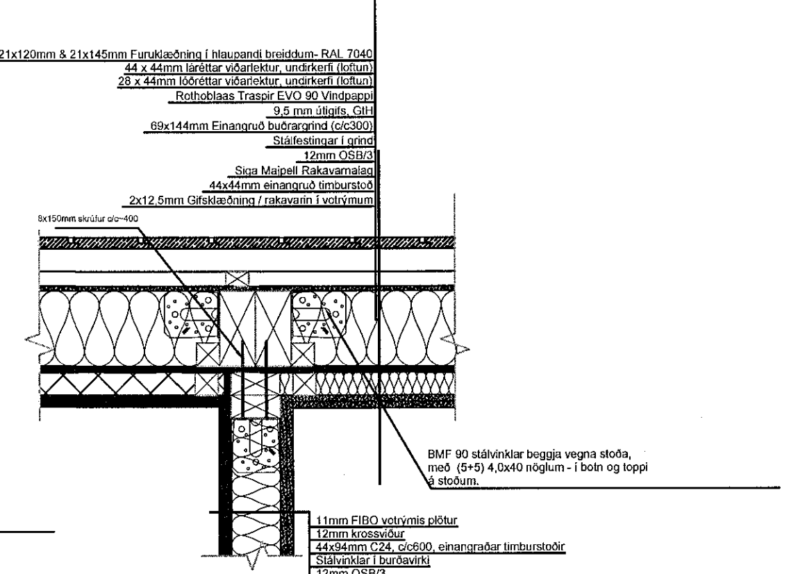
TENING INN- OG ÚTVEGGJAR, KENNISNIÐ, 1:10
