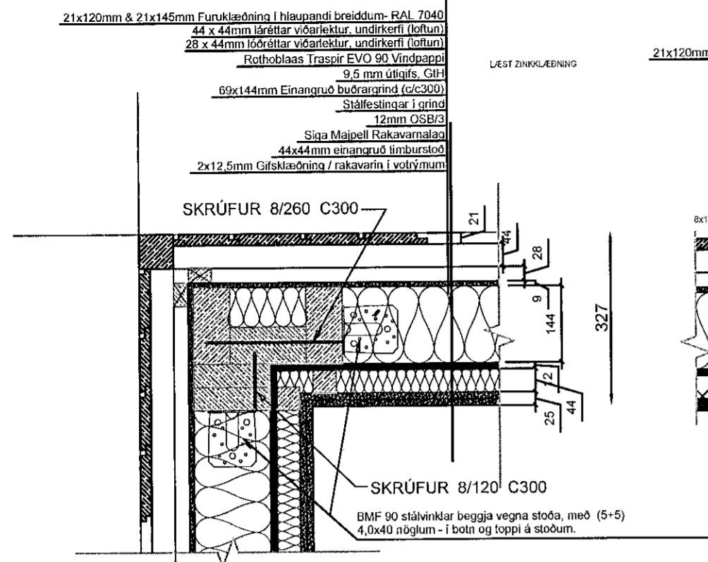
FRÁGANGUR Á ÚTHORNI, KENNISNIÐ, 1:10
