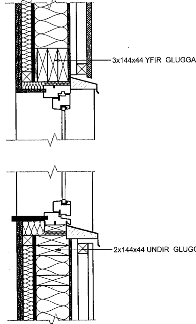
FRÁGANGUR YFIR OG UNDIR GLUGGA, KENNISNIÐ, 1:10
