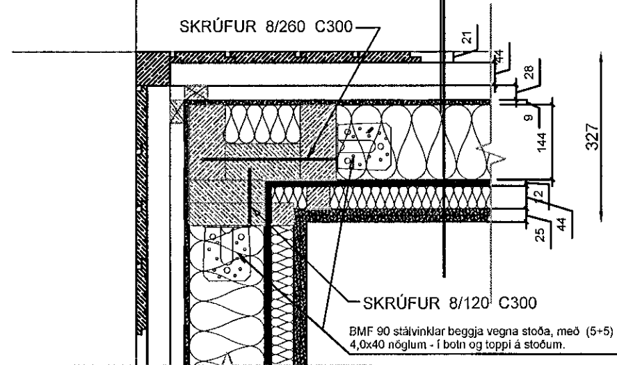
FRÁGANGUR Á ÚTHORNI, KENNISNIÐ, 1:10
