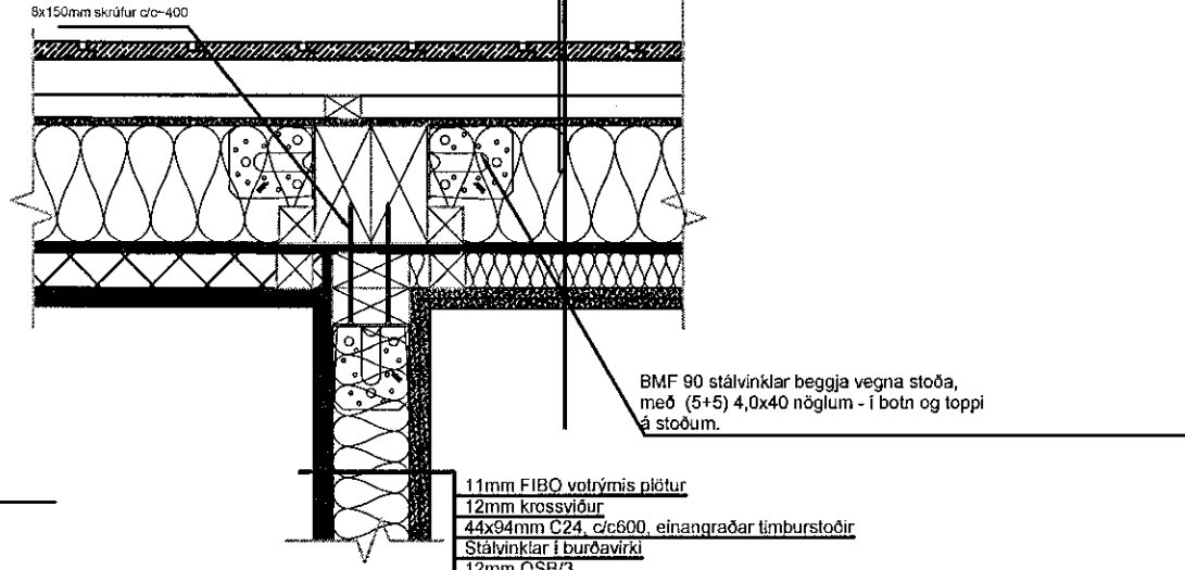
TENING INN- OG ÚTVEGGJAR, KENNISNIÐ, 1:10
