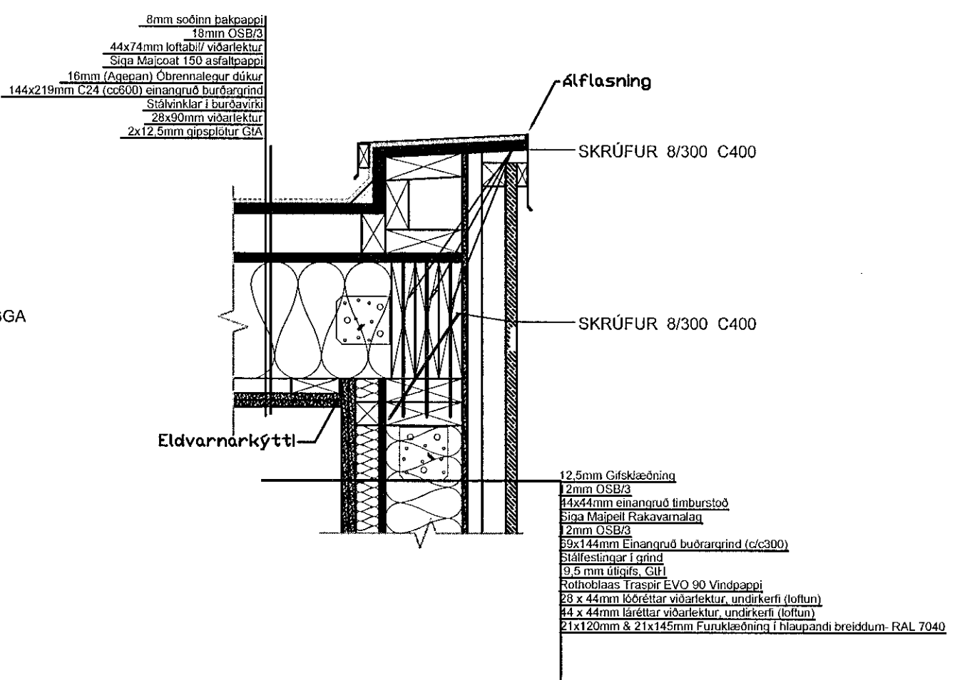
TENING ÞAKS OG ÚTVEGGJAR, KENNISNIÐ, 1:10
