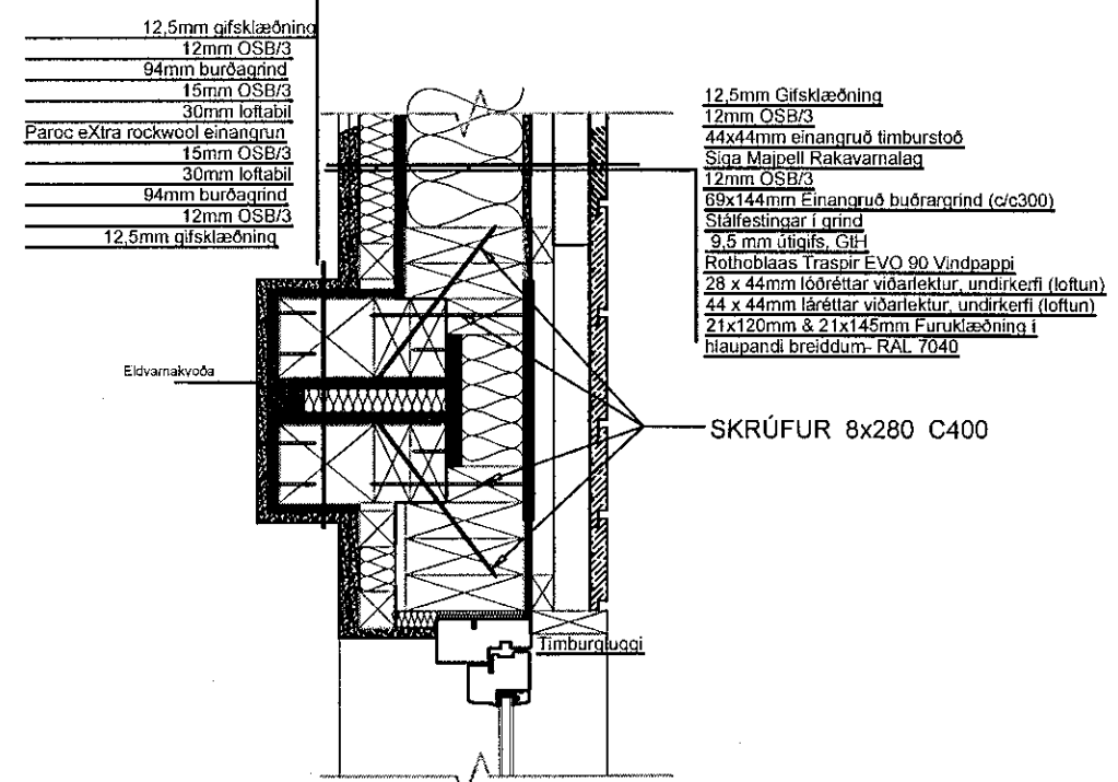
TENING TVEGGJA EINGA, KENNISNIÐ, 1:10
