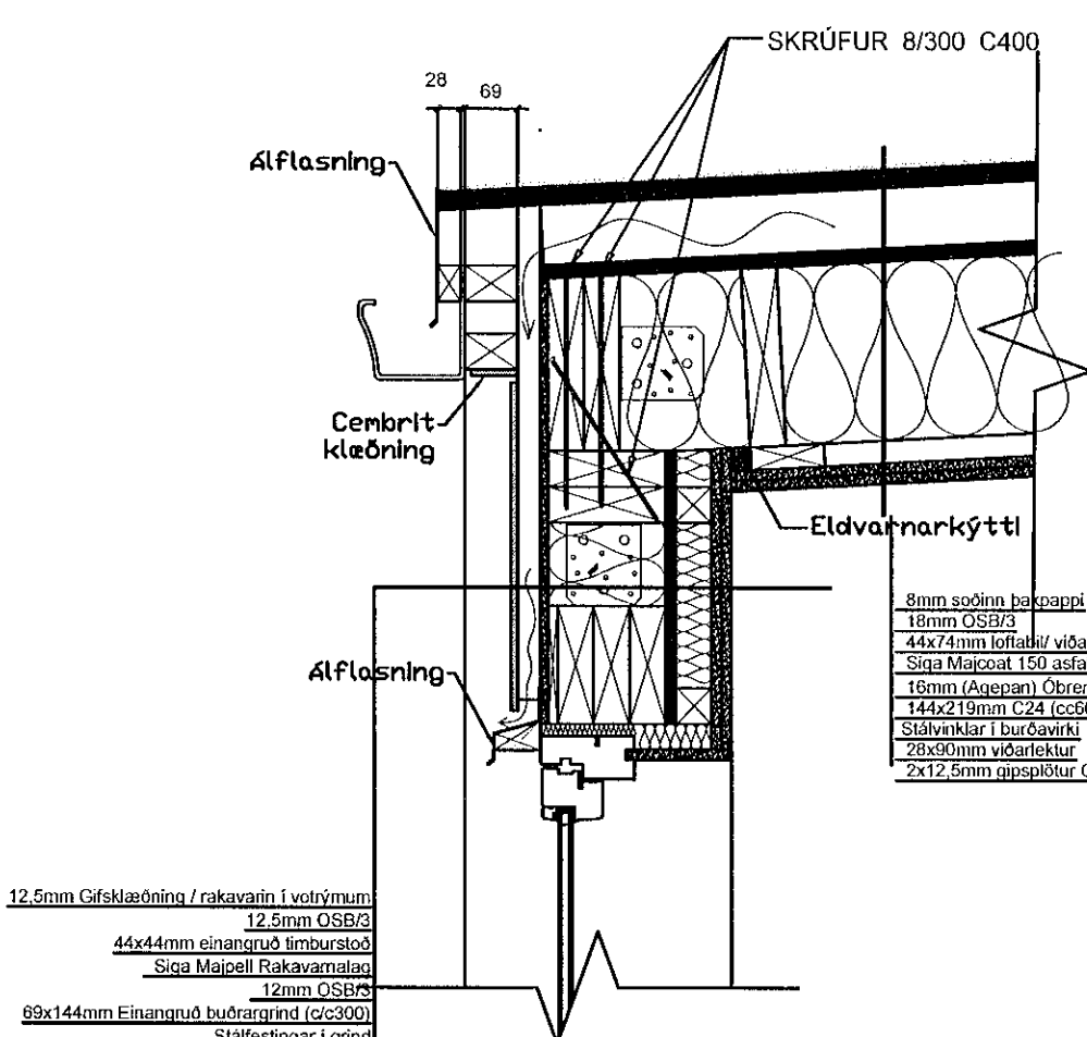
TENING ÞAKS OG ÚTVEGGJAR, KENNISNIÐ, 1:10
