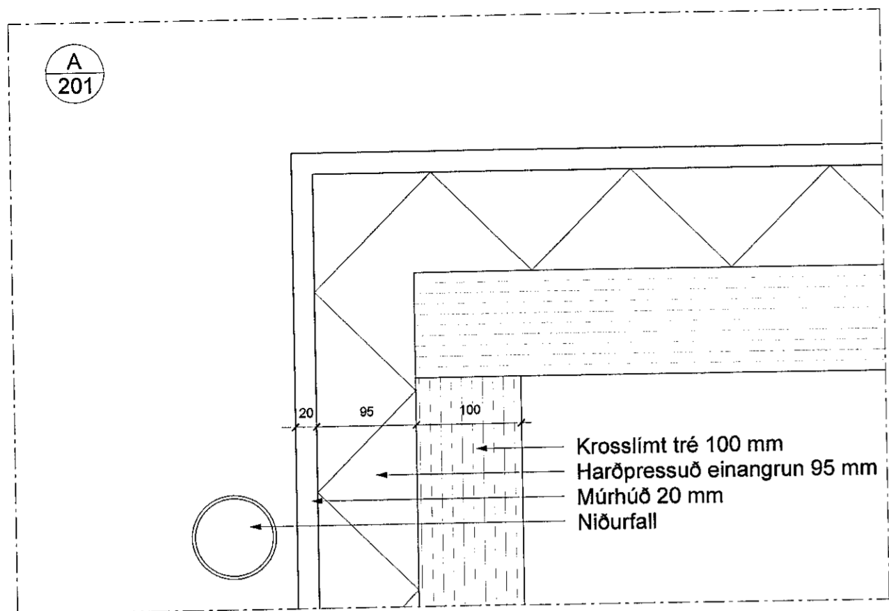
Lárétt deili A 1:5
