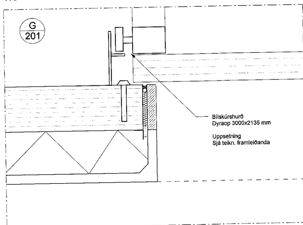
Lárétt deili G 1:5
