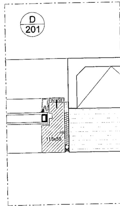
Lárétt deili D 1:5
