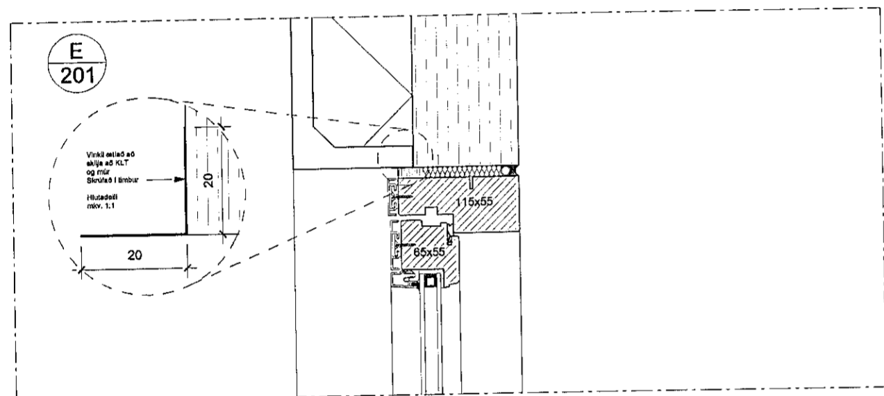
Lárétt deili E 1:5
