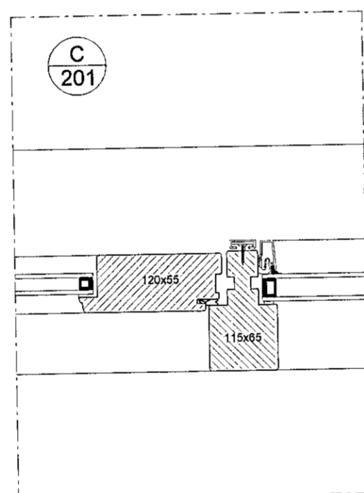
Lárétt deili C 1:5
