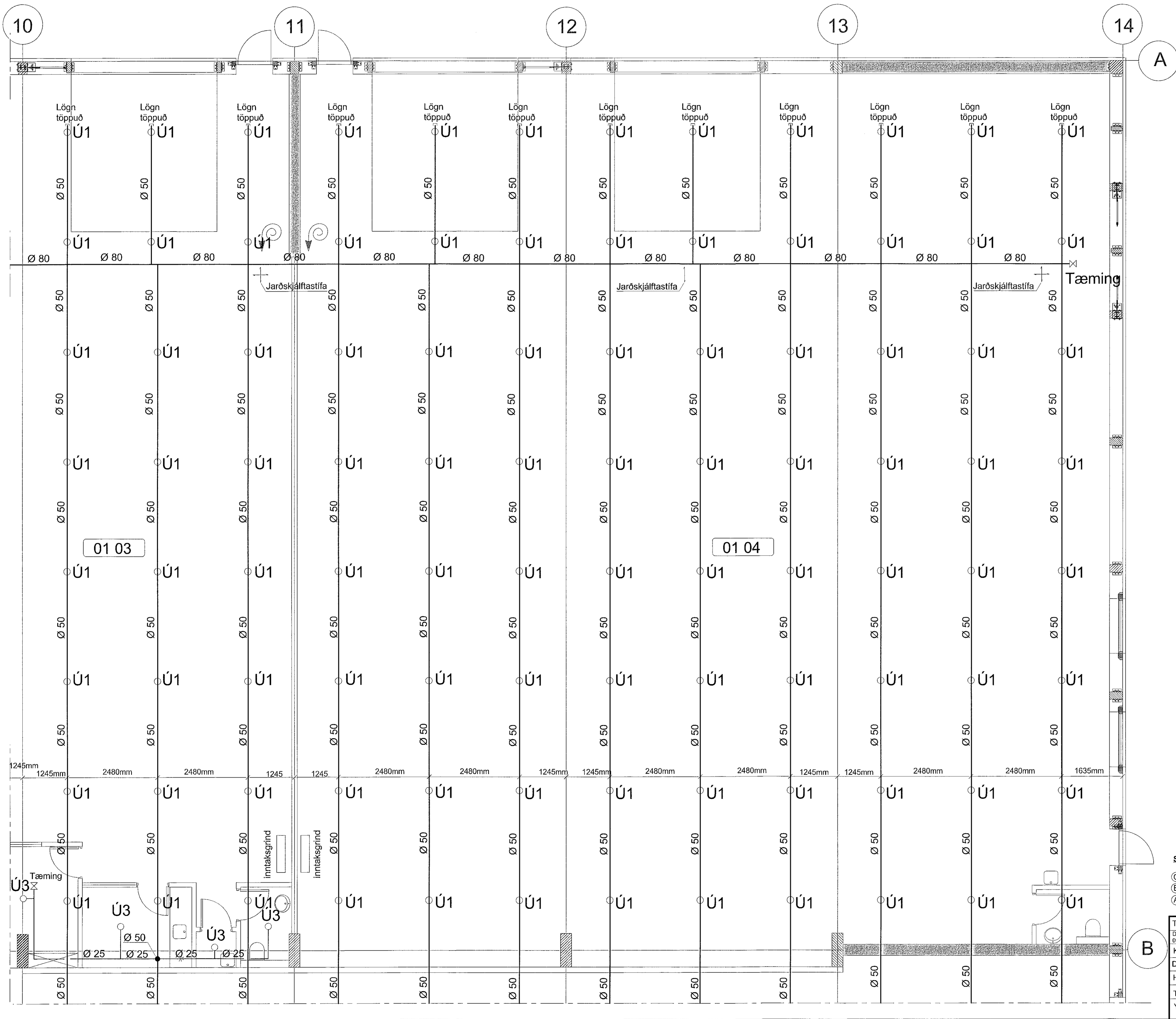
LYKILMYND 1:1000
